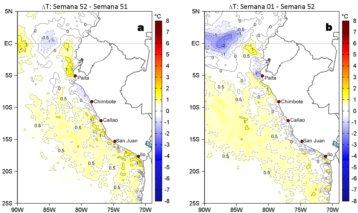
Figura 4. Variación semanal de la TSM ( ^{\circ}\text{C} ) en el océano Pacífico tropical oriental entre: a) quincuagésima segunda (22 - 28 de diciembre) y quincuagésima primera (15 - 21 de diciembre) semana de 2025 y b) primera (29 de diciembre - 04 de enero) semana de 2026 y quincuagésima segunda (22 - 28 de diciembre) semana de 2025. Los mapas, que indican el grado de calentamiento o enfriamiento de una semana a otra, provienen de OSTIA-UKMO-L4-GLOB-v2.0 (UK Met Office, 2012; Donlon et al, 2012).
