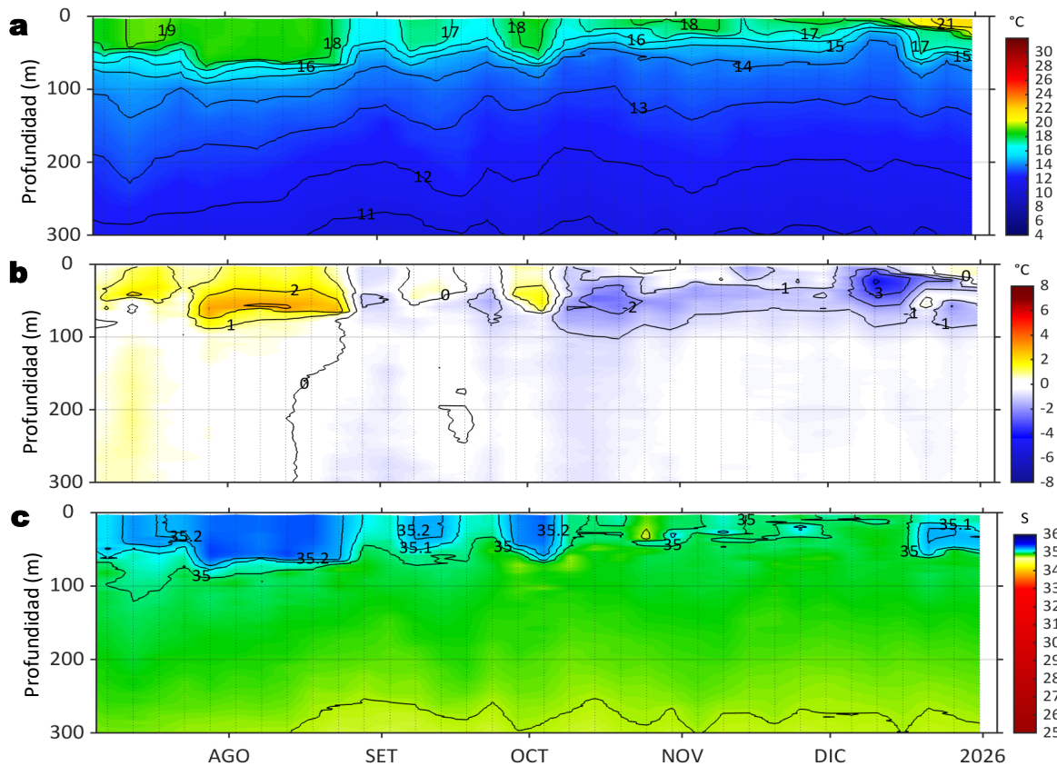
Figura 7. Diagrama Hovmöller de: a) Temperatura del mar (°C), b) Anomalías térmicas (°C) y c) Salinidad del mar registrados por el perfilador ARGO No. 3903004, a 82 mn (12,83°S y 78,22°W) frente a Callao el día 31 de diciembre del 2025. Las anomalías térmicas se calcularon de acuerdo a Domínguez et al (2023). Los puntos en la columna de agua indican los días en que el perfilador registró información. Datos: ARGO.
