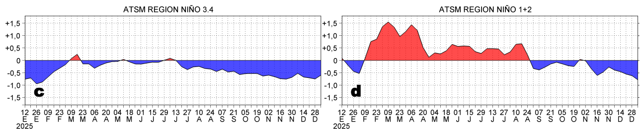
Figura 1. Anomalías promedio de la temperatura superficial del mar (TSM, °C) en el océano Pacífico tropical del 22 al 28 de diciembre del 2025 (a) y del 29 de diciembre del 2025 al 04 de enero del 2026 (b), así como la variación del promedio semanal durante el último año para la región Niño 3.4 (c) y la región Niño 1+2 (d). Las regiones Niño 3.4 y Niño 1+2 en los sectores central y oriental del océano, respectivamente, están delimitadas con una línea de color gris. Datos: OSTIA-UKMO-L4-GLOB-v2.0 (UK Met Office, 2012; Donlon et al, 2012). Climatología: 1991-2020.
