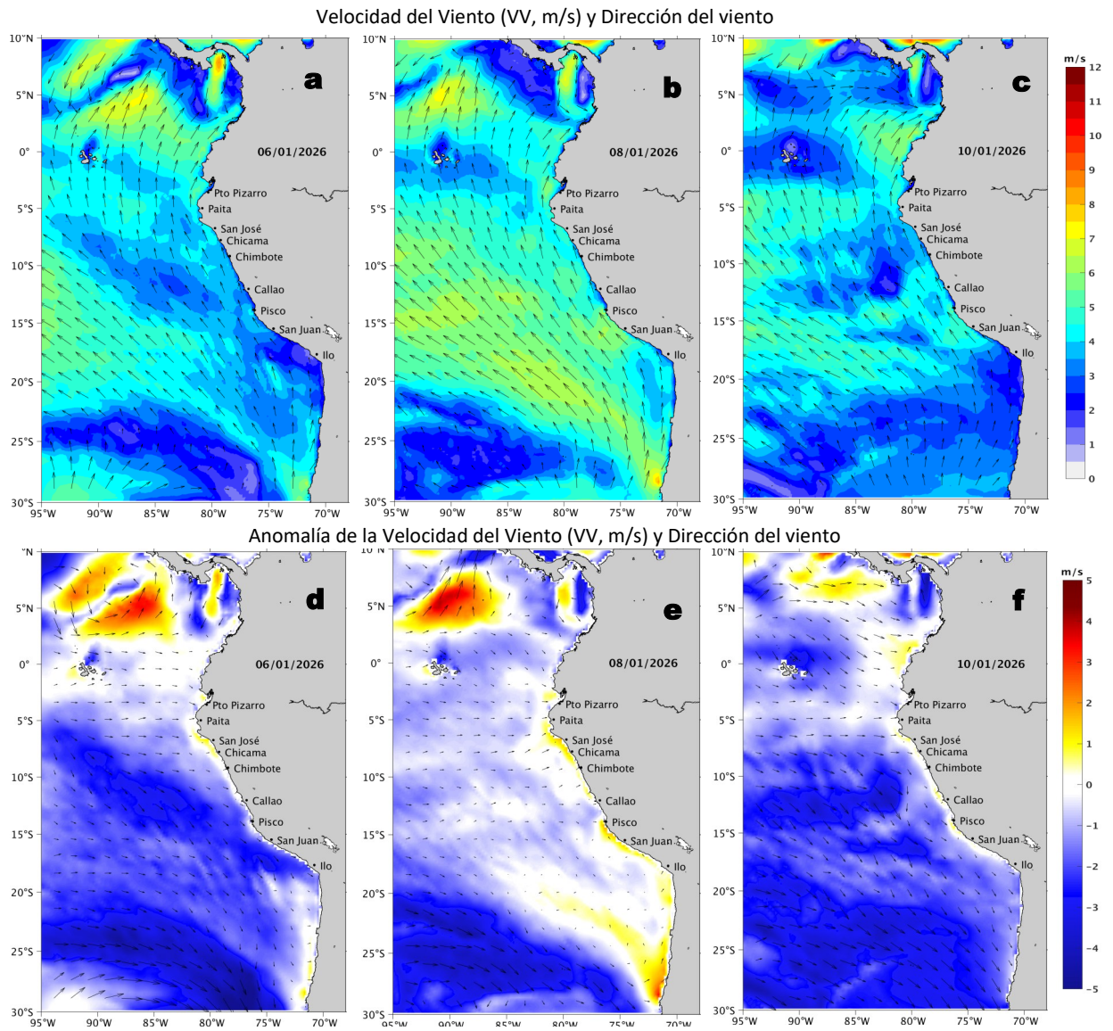
Figura 10. Distribución espacial del pronóstico de la velocidad del viento (VV, m/s) y dirección del viento ( ^{\circ} ), así como para sus anomalías para los días a) 06, b) 08 y c) 10 de enero de 2026, frente a la costa sudamericana entre Centroamérica y la costa norte de Chile. Fuente: Modelo Climate Forecast System (GFS) de la NOAA. Climatología: 2000-2020.
