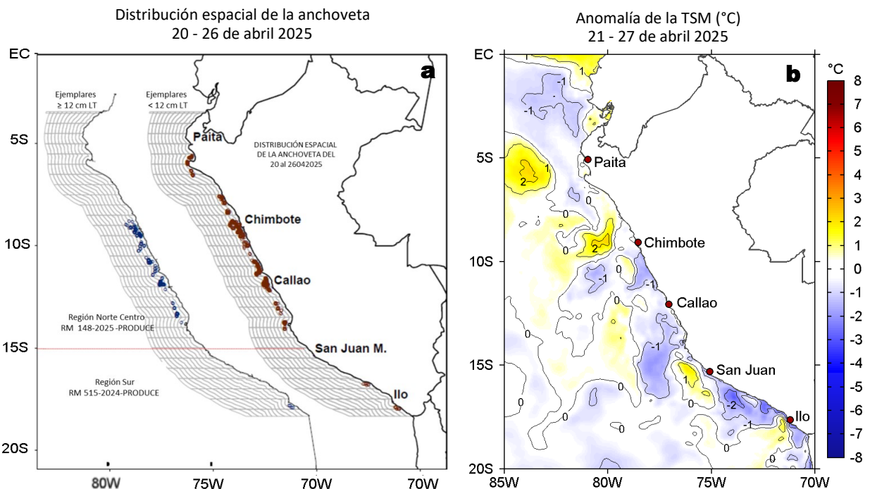
Figura 9. a) Distribución de la anchoveta según porcentaje de juveniles por región y su relación con b) las anomalías térmicas ( ^{\circ}\text{C} ) para la semana del 21 al 27 de abril de 2025. Datos: OSTIA-UKMO-L4-GLOB-v2.0 (UK Met Office, 2012; Donlon et al, 2012). Las anomalías térmicas se calcularon con respecto de la climatología para el período 1991-2020.
