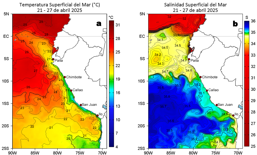
Figura 3. Distribución espacial promedio de la: a) Temperatura superficial del Mar (TSM, °C) y b) Salinidad superficial del mar (SSM) del 21 al 27 de abril del 2025. Datos: OSTIA-UKMO-L4-GLOB-v2.0 (UK Met Office, 2012; Donlon et al, 2012) para (a) y del GLOBAL_ANALYSISFORECAST_PHY_001_024 (Lellouche, J. M. et al, 2013) para (b).
