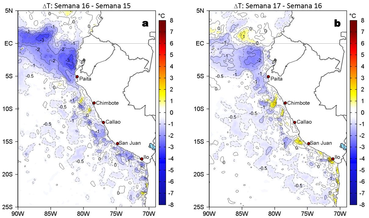
Figura 4. Variación semanal de la TSM (°C) en el océano Pacífico tropical oriental entre: a) décima sexta (14 - 20 de abril) y décima quinta (07 - 13 de abril) semana del 2025 y b) décima séptima (21 - 27 de abril) y décima sexta (14 - 20 de abril) semana del 2025. Los mapas, que indican el grado de calentamiento o enfriamiento de una semana a otra, provienen de OSTIA-UKMO-L4-GLOB-v2.0 (UK Met Office, 2012; Donlon et al, 2012).
