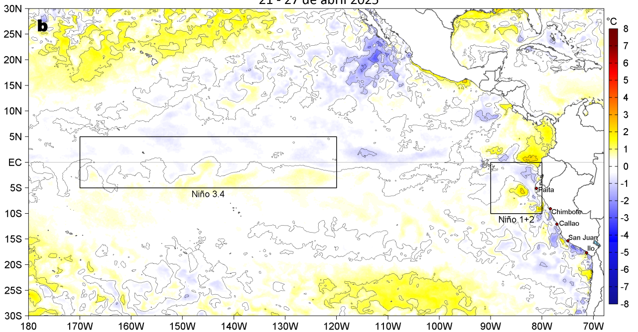
Anomalías de la Temperatura Superficial del Mar (°C) 21 - 27 de abril 2025
