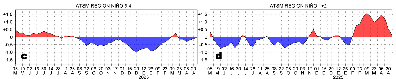
Figura 1. Anomalías promedio de la temperatura superficial del mar (TSM, °C) en el océano Pacífico tropical del 14 al 20 de abril (a) y del 21 al 27 de abril (b) del 2025, así como la variación del promedio semanal durante el último año para la región Niño 3.4 (c) y la región Niño 1+2 (d). Las regiones Niño 3.4 y Niño 1+2 en los sectores central y oriental del océano, respectivamente, están delimitadas con una línea de color gris. Datos: OSTIA-UKMO-L4-GLOB-v2.0 (UK Met Office, 2012; Donlon et al, 2012). Climatología: 1991-2020.
