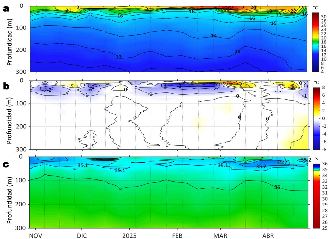
Figura 7. Diagrama Hovmöller de: a) Temperatura del mar (°C), b) Anomalías térmicas (°C) y c) Salinidad del mar registrados por el perfilador ARGO No. 3902381 a 79 mn (10,92°S y 78,57°W) frente a Huacho, el día 27 de abril del 2025. Las anomalías de la temperatura del agua se calcularon de acuerdo a Domínguez et al (2023). Los puntos en la columna de agua indican los días en que el perfilador registró información. Datos: ARGO.
