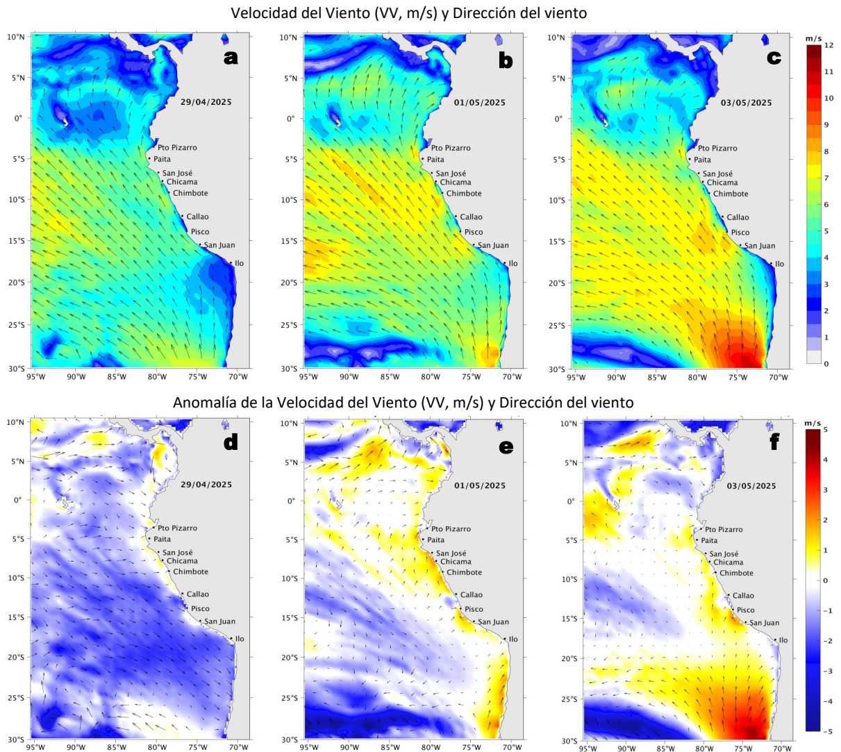
Figura 10. Distribución espacial del pronóstico de la velocidad del viento (VV, m/s) y dirección del viento ( ^{\circ} ), así como para sus anomalías para los días a) 29 de abril, b) 01 y c) 03 de mayo de 2025, frente a la costa sudamericana entre Centroamérica y la costa norte de Chile. Fuente: Modelo Climate Forecast System (GFS) de la NOAA. Climatología: 2000-2020.
