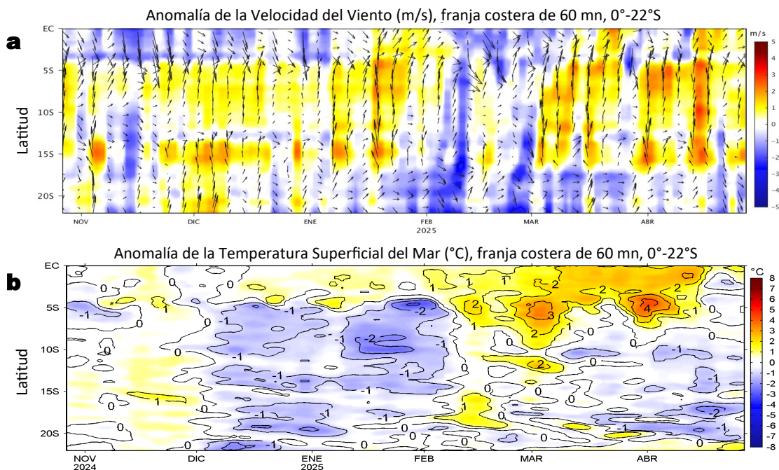
Figura 6. Evolución de las anomalías diarias de: a) Velocidad del viento (m/s) y b) TSM (°C) de octubre del 2024 al 27 de abril del 2025. Datos: GFS para (a) y OSTIA-UKMO-L4-GLOB-v2.0 para (b). Las anomalías fueron calculadas para una franja de 60 mn adyacente a la costa entre el ecuador geográfico y 22°S según los promedios diarios de 2000-2014 para (a) y de 1991-2020 para (b). La barra de colores a la derecha muestra la escala de las anomalías en cada caso.
