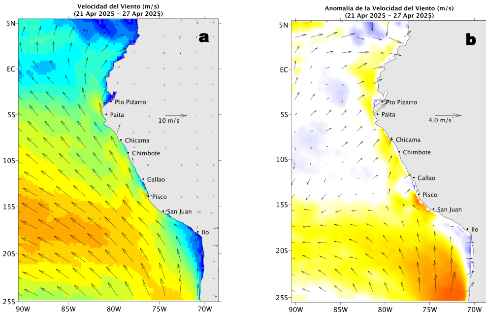
Figura 2. Distribución espacial promedio de: a) la velocidad (m/s) y dirección del viento (°) y b) anomalías de la velocidad (m/s) y dirección del viento (°) frente a la costa peruana del 21 al 27 de abril del 2025. La velocidad del viento y su anomalía se presentan en matices de colores. La dirección del viento y su anomalía se presentan con flechas. Fuente de los datos: GFS. Climatología: QuikSCAT-ASCAT 2000-2014.
