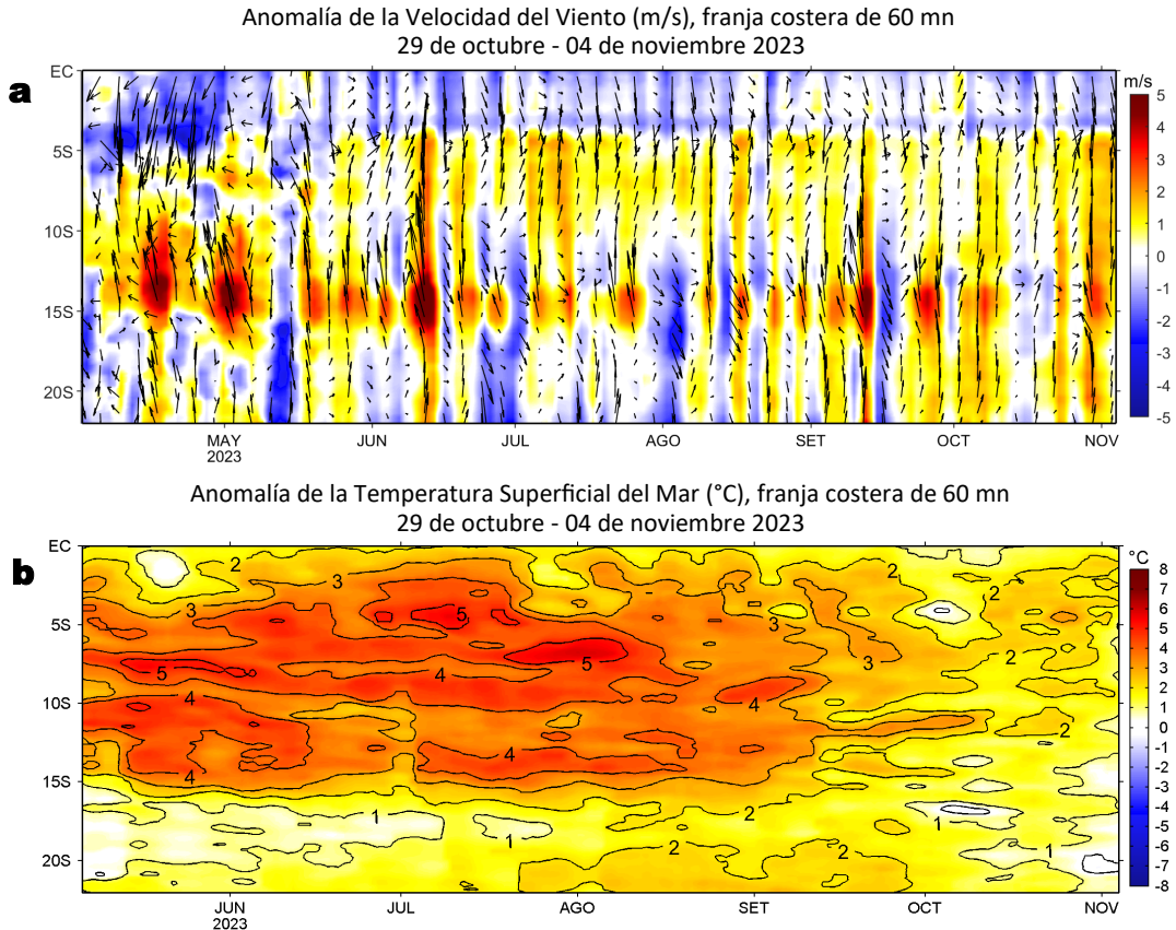
Figura 5. Evolución de las anomalías diarias de: a) Velocidad del viento (m/s) y b) Temperatura superficial del mar (°C) para el último semestre, actualizado al 04 de noviembre de 2023. Datos: de IFREMER/CERSAT para (a) y de OSTIA-UKMO-L4-GLOB-v2.0 para (b). Las anomalías fueron calculadas para una franja de 60 mn adyacente a la costa entre el ecuador geográfico y 22°S según los promedios climatológicos diarios de 2000-2014 para (a) y de 1991-2020 para (b). La barra de colores a la derecha muestra la escala de las anomalías en cada caso.
