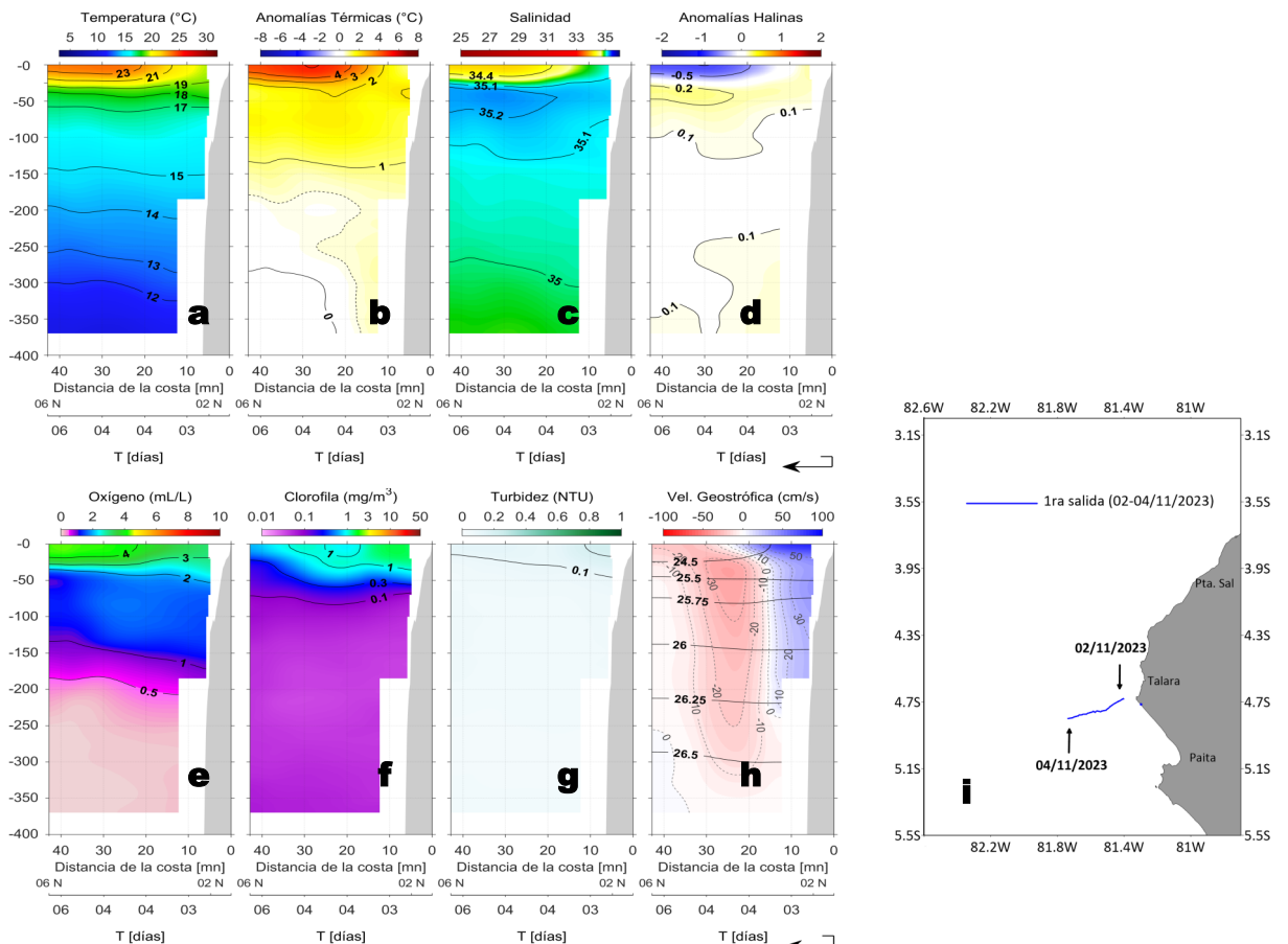
Figura 7. Estructura de: a) Temperatura del agua de mar (°C), b) Anomalías térmicas (°C), c) Salinidad, d) Anomalías halinas, e) Oxígeno (mL/L), f) Clorofila "a" (mg/m 3 ), g) Turbidez (NTU), h) Velocidades geostróficas (cm/s) e i) Recorrido del glider Nazca del 02 al 04 de noviembre del 2023.
