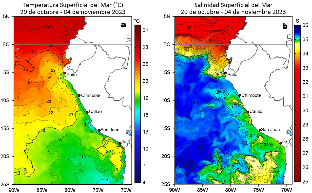
Figura 2. Distribución espacial promedio de: a) TSM (°C) y b) Salinidad superficial del mar (SSM) para la semana del 29 de octubre al 04 de noviembre 2023. Datos: OSTIA-UKMO-L4-GLOB-v2.0 (UK Met Office, 2012; Donlon et al, 2012) disponible en https://podaac.jpl.nasa.gov/dataset/OSTIA-UKMO-L4-GLOB-v2.0 para (a) y del GLOBAL_ANALYSISFORECAST_PHY_001_024 (Lellouche, J. M. et al, 2013) disponible en https://data.marine.copernicus.eu/product/GLOBAL_ANALYSISFORECAST_PHY_001_024/description para (b). Las escalas de colores se presentan a la derecha de cada gráfico.
