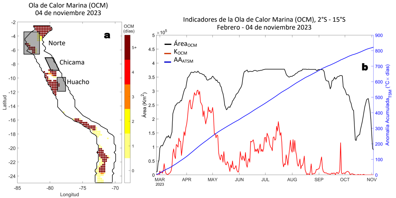
Figura 4. a) Extensión de la ola de calor marina (OCM) entre los 2 y 15°S dentro de la franja de 150 mn frente a la costa desde su inicio a fines de febrero del 2023 al 04 de noviembre; la escala de color indica el número de días en los cuales la TSM ha superado el percentil 90 de los datos diarios históricos, usando el período 1982-2011 como referencia (Pietri et al., 2021). b) Series de tiempo de indicadores de la OCM para la zona entre los 2 y 15°S y dentro de las 150 mn: área de la OCM ( A_{OCM} , Km^2 ); área de la OCM donde la ATSM > +4 °C ( K_{OCM} , Km^2 ); y anomalía acumulada ( AA_{ATSM} ; °C x días). Desde su inicio, la OCM acumuló una anomalía de TSM de 822,43 °C días totalizando 252 días de duración. Fuente: OISST 2.1; procesamiento: IMARPE/AFIOF.
