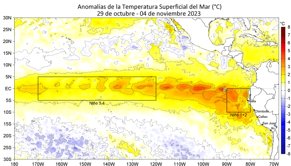
Figura 1. Anomalías promedio de la temperatura superficial del mar (TSM, °C) en el océano Pacífico tropical para la semana del 29 de octubre al 04 de noviembre de 2023. Las regiones Niño 3.4 y Niño 1+2 en los sectores central y oriental del océano, respectivamente, están delimitadas con una línea de color gris. Datos: OSTIA-UKMO-L4-GLOB-v2.0 (UK Met Office, 2012; Donlon et al, 2012) disponible en https://podaac.jpl.nasa.gov/dataset/OSTIA-UKMO-L4-GLOB-v2.0 . Las anomalías se calcularon con respecto de la climatología para el periodo 1991-2020 (Quispe, in prep. ).
