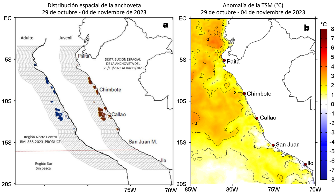
Figura 10. a) Distribución de la anchoveta según porcentaje de juveniles por región y su relación con b) las anomalías térmicas ( ^{\circ}\text{C} ) para la semana del 29 de octubre al 04 de noviembre de 2023. Datos: OSTIA-UKMO-L4-GLOB-v2.0 (UK Met Office, 2012; Donlon et al, 2012) disponible en https://podaac.jpl.nasa.gov/dataset/OSTIA-UKMO-L4-GLOB-v2.0 . Las anomalías térmicas se calcularon con respecto de la climatología para el período 1991-2020.
