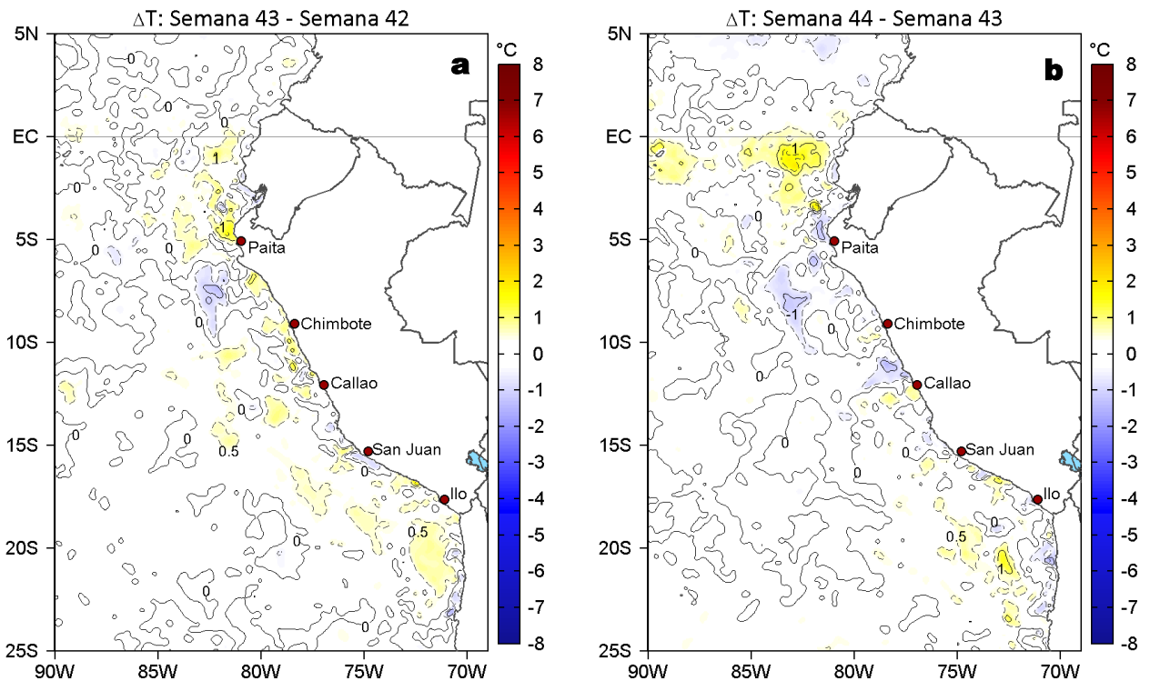
Figura 3. Variación semanal de la TSM (°C) en el océano Pacífico tropical oriental entre: a) cuadragésima tercera (22-28 de octubre) y cuadragésima segunda (15-21 de octubre) semana de 2023 y b) cuadragésima cuarta (29 de octubre - 04 de noviembre) y cuadragésima tercera (22-28 de octubre) semana de 2023. Los mapas, que indican el grado de calentamiento o enfriamiento de una semana a otra, provienen de OSTIA-UKMO-L4-GLOB-v2.0 (UK Met Office, 2012; Donlon et al, 2012). La barra de colores a la derecha muestra la diferencia de la temperatura entre la presente y la semana previa.
