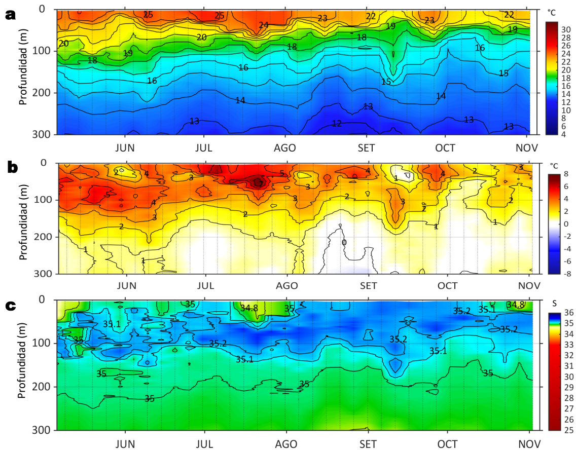
Figura 8. Diagrama Hovmöller de: a) Temperatura del mar (°C), b) Anomalías térmicas (°C) y c) Salinidad del mar, perfilador ARGO No. 6903002 localizado a 95 mn (3,96°S, 82,64°W) frente a Tumbes el 02 de noviembre de 2023. Las anomalías de la temperatura del agua se calcularon de acuerdo a Domínguez et al., 2023. Los puntos en la columna de agua indican los días en que el perfilador registró información. Datos: ARGO.
