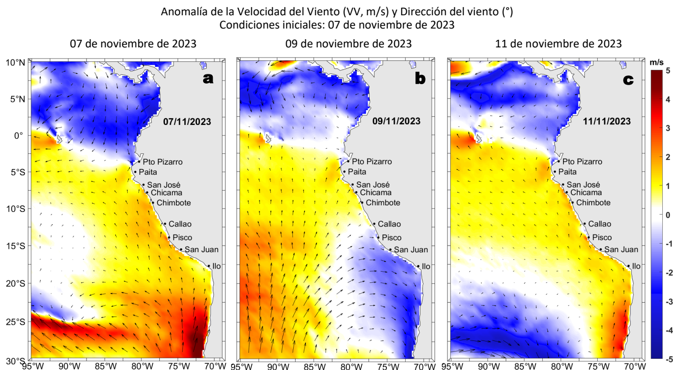
Figura 11. Distribución espacial del pronóstico de las anomalías de la Velocidad del Viento (VV, m/s) y dirección del viento ( ^{\circ} ) para los días a) 07, b) 09 y c) 11 de noviembre de 2023, frente a la costa entre Panamá y Chile. Fuente: Modelo Climate Forecast System (GFS) de la NOAA.
