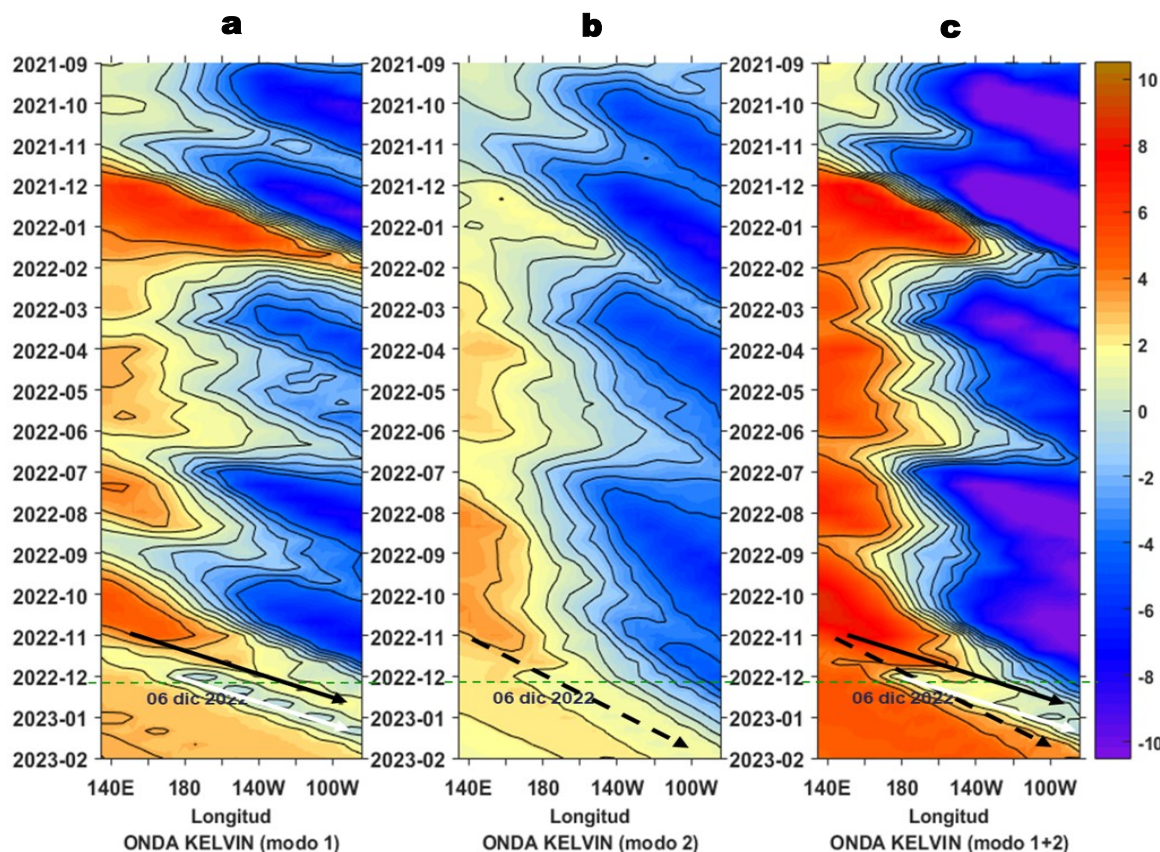
Figura 7. Diagramas Hovmöller longitudud-tiempo de las Ondas Kelvin Ecuatoriales en el Océano Pacífico Ecuatorial entre 130°E y 95°W forzado con anomalías del esfuerzo del viento (N/m 2 ) del NCEP (Kalnay et al. 1996) de acuerdo con la metodología de Illig et al. (2004) y Dewitte et al. (2002): a) Modo 1, b) Modo 2 y c) Modos 1+2. La línea discontinua horizontal de color verde indica el inicio del pronóstico con anomalías del esfuerzo del viento igual a cero. Los valores negativos corresponden a ondas Kelvin de afloramiento “frías” (flechas blancas). Datos de modelo: Laboratorio de Modelado Oceanográfico Ecosistemico y de Cambio Climático (LMOECC).
