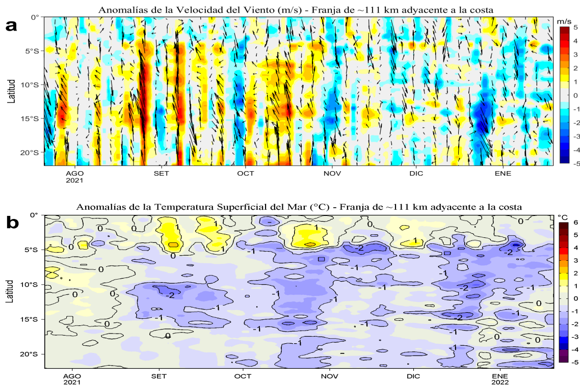
Figura 4. Evolución de las anomalías diarias de: a) Velocidad del viento (m/s) y b) Temperatura superficial del mar (°C) para el último semestre, actualizado al 19 y 20 de enero de 2022, respectivamente. Datos: de IFREMER/CERSAT para (a) y de OSTIA-UKMO-L4-GLOB-v2.0 para (b). Las anomalías fueron calculadas para una franja de 111 km adyacente a la costa entre el ecuador geográfico y 22°S según los promedios climatológicos diarios de 2000-2014 para (a) y de 2007-2016 para (b). La barra de colores a la derecha muestra la escala de las anomalías en cada caso.
