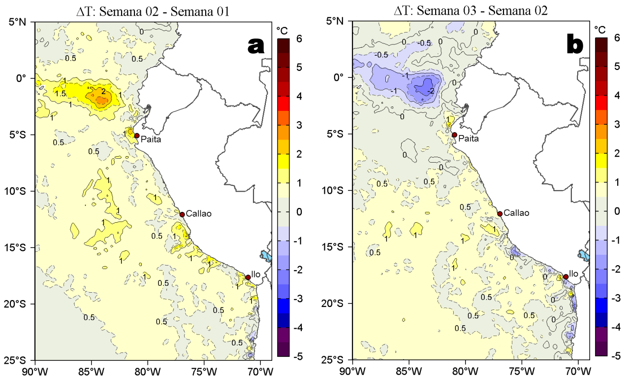
Figura 3. Variación semanal de la temperatura superficial del mar (°C) en el océano Pacífico tropical oriental entre: a) segunda (07-13 de enero) y primera (01-06 de enero) semana de 2022 y b) tercera (14-20 de enero) y segunda (07-13 de enero) semana de 2022. Los mapas, que indican el grado de calentamiento o enfriamiento de una semana a otra, provienen de OSTIA-UKMO-L4-GLOB-v2.0 (UK Met Office, 2012; Donlon et al, 2012). La barra de colores a la derecha muestra la diferencia de la temperatura entre la presente y la semana previa.
