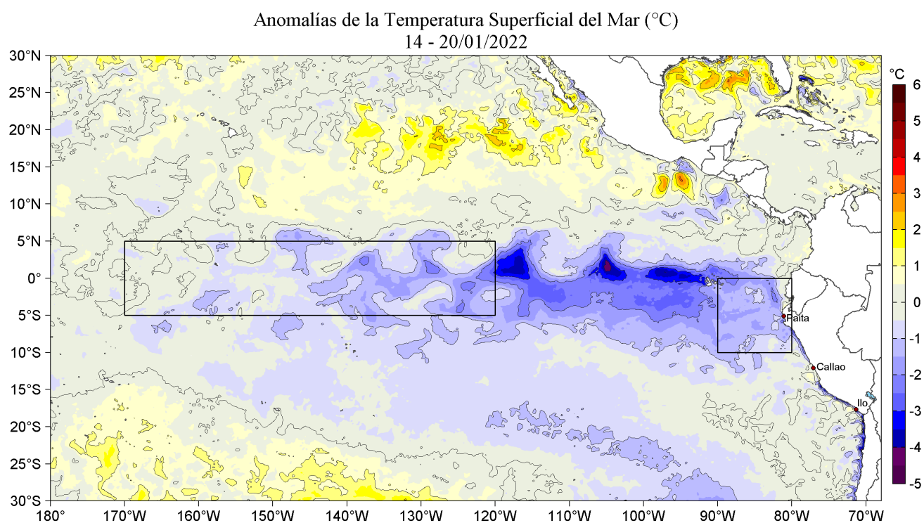
Figura 1. Anomalías promedio de la Temperatura superficial del mar (°C) en el océano Pacífico tropical para la semana del 14 al 20 de enero de 2022. Las regiones Niño 3.4 y Niño 1+2 en los sectores central y oriental del océano, respectivamente están delimitadas con una línea de color gris. Datos: OSTIA-UKMO-L4-GLOB-v2.0 (UK Met Office, 2012; Donlon et al, 2012) disponible en https://podaac.jpl.nasa.gov/dataset/OSTIA-UKMO-L4-GLOB-v2.0 . Las anomalías se calcularon con respecto de la climatología para el periodo 2007-2016.
