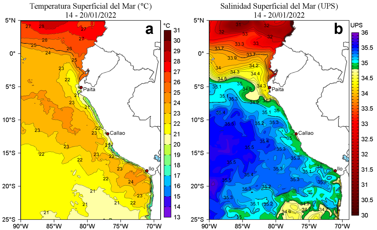
Figura 2. Distribución espacial promedio de: a) Temperatura (TSM, °C) y b) Salinidad superficial del mar (SSM) para la semana del 14 al 20 de enero de 2022, en el océano Pacífico oriental. Datos: OSTIA-UKMO-L4-GLOB-v2.0 (UK Met Office, 2012; Donlon et al, 2012) disponible en https://podaac.jpl.nasa.gov/dataset/OSTIA-UKMO-L4-GLOB-v2.0 para (a) y del GLOBAL_ANALYSIS_FORECAST_PHY_001_024 (Lellouche, J. M. et al, 2013) disponible en http://marine.copernicus.eu/services-portfolio/access-to-products/?option=com_csw&view=details&product_id=GLOBAL_ANALYSIS_FORECAST_PHY_001_024 para (b). Las escalas de colores se presentan a la derecha de cada gráfico.
