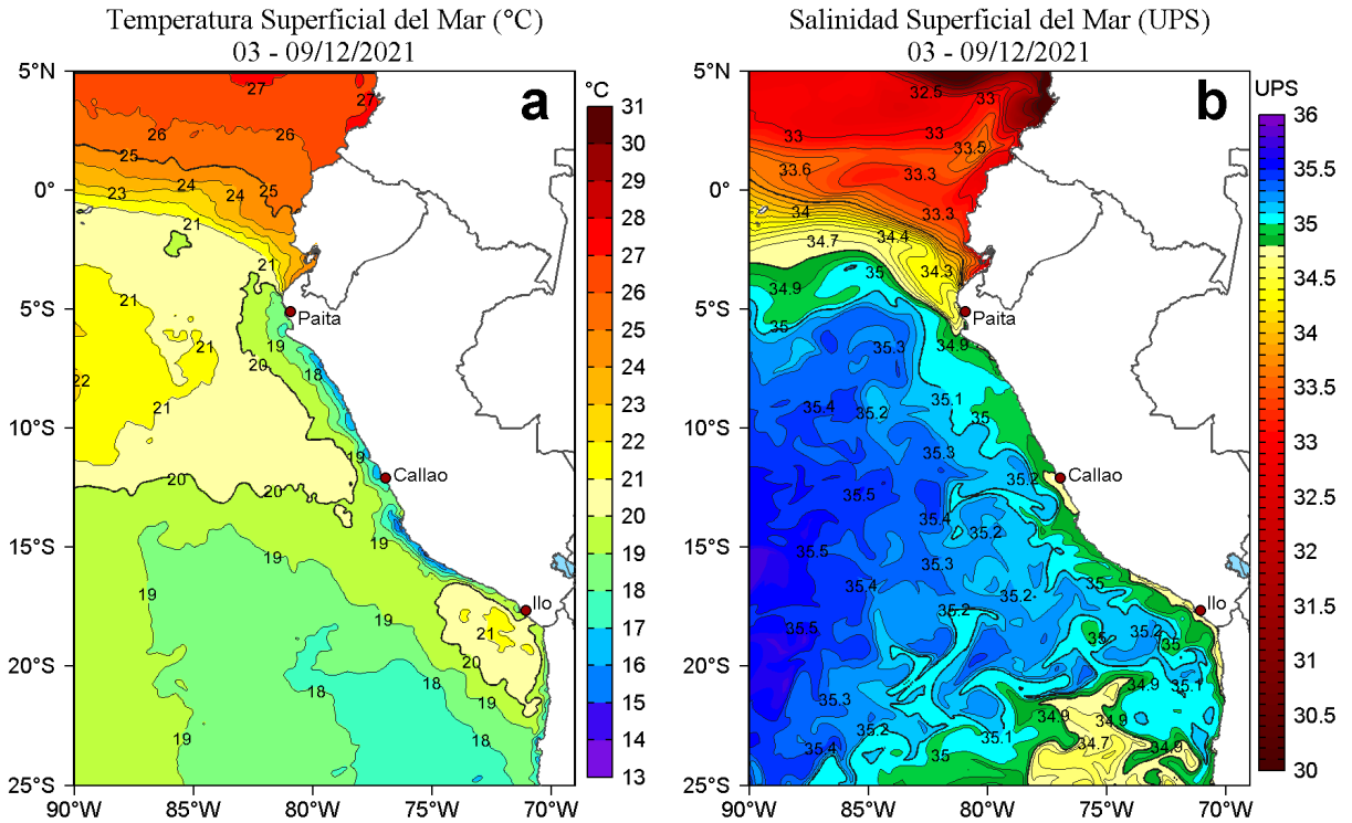
Figura 2. Distribución espacial promedio de: a) Temperatura (TSM, °C) y b) Salinidad superficial del mar (SSM) para la semana del 03 al 09 de diciembre de 2021, en el océano Pacífico oriental. Datos: OSTIA-UKMO-L4-GLOB-v2.0 (UK Met Office, 2012; Donlon et al, 2012) disponible en https://podaac.jpl.nasa.gov/dataset/OSTIA-UKMO-L4-GLOB-v2.0 para (a) y del GLOBAL ANALYSIS FORECAST PHY 001 024 (Lellouche, J. M. et al, 2013) disponible en http://marine.copernicus.eu/services-portfolio/access-to-products/?option=com_csw&view=details&product_id=GLOBAL_ANALYSIS_FORECAST_PHY_001_024 para (b). Las escalas de colores se presentan a la derecha de cada gráfico.
