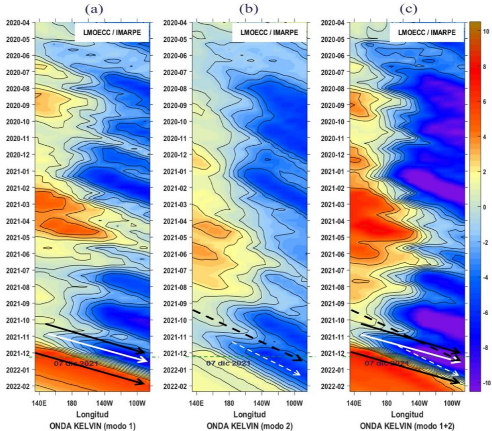
Figura 8. Diagramas Hovmöller longitud-tiempo de las Ondas Kelvin Ecuatoriales en el Océano Pacífico Ecuatorial entre 130°E y 95°W forzado con anomalías del esfuerzo del viento ( N/m^2 ) del NCEP (Kalnay et al. 1996) de acuerdo con la metodología de Illig et al. (2004) y Dewitte et al. (2002): a) Modo 1, b) Modo 2 y c) Modos 1+2. La línea discontinua horizontal de color verde indica el inicio del pronóstico con anomalías del esfuerzo del viento igual a cero. Los valores negativos corresponden a ondas Kelvin de afloramiento “frías” (flechas blancas).
