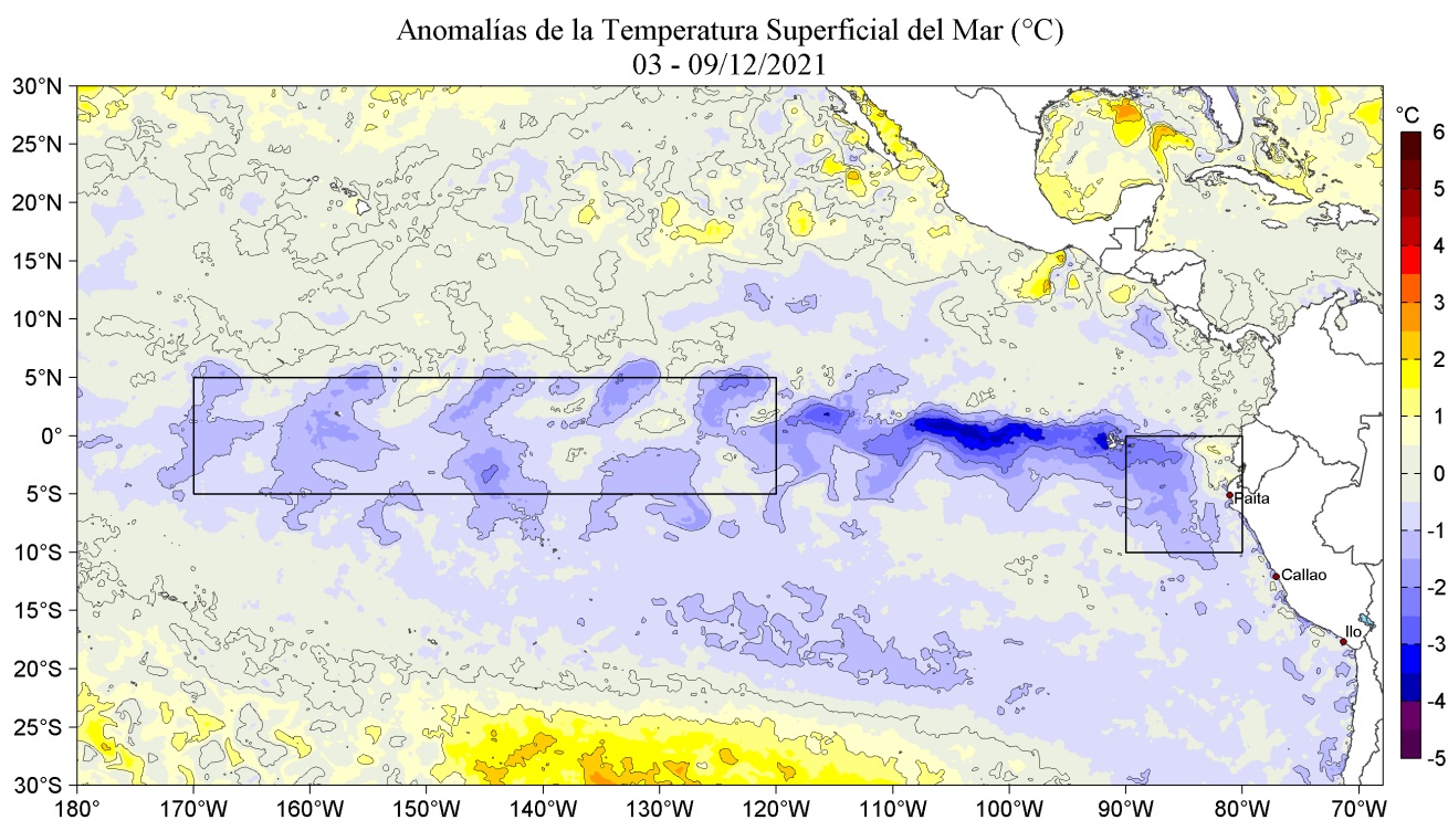
Figura 1. Anomalías promedio de la Temperatura superficial del mar (°C) en el océano Pacífico tropical para la semana del 03 al 09 de diciembre de 2021. Las regiones Niño 3.4 y Niño 1+2 en los sectores central y oriental del océano, respectivamente están delimitadas con una línea de color gris. Datos: OSTIA-UKMO-L4-GLOB-v2.0 (UK Met Office, 2012; Donlon et al, 2012) disponible en https://podaac.jpl.nasa.gov/dataset/OSTIA-UKMO-L4-GLOB-v2.0 . Las anomalías se calcularon con respecto de la climatología para el período 2007-2016.
