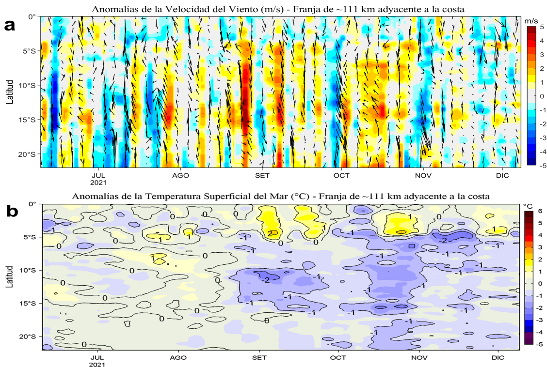
Figura 4. Evolución de las anomalías diarias de: a) Velocidad del viento (m/s) y b) Temperatura superficial del mar (°C) para el último semestre, actualizado al 08 y 09 de diciembre de 2021, respectivamente. Datos: de IFREMER/CERSAT para (a) y de OSTIA-UKMO-L4-GLOB-v2.0 para (b). Las anomalías fueron calculadas para una franja de 111 km adyacente a la costa entre el ecuador geográfico y 22°S según los promedios climatológicos diarios de 2000-2014 para (a) y de 2007-2016 para (b). La barra de colores a la derecha muestra la escala de las anomalías en cada caso.
