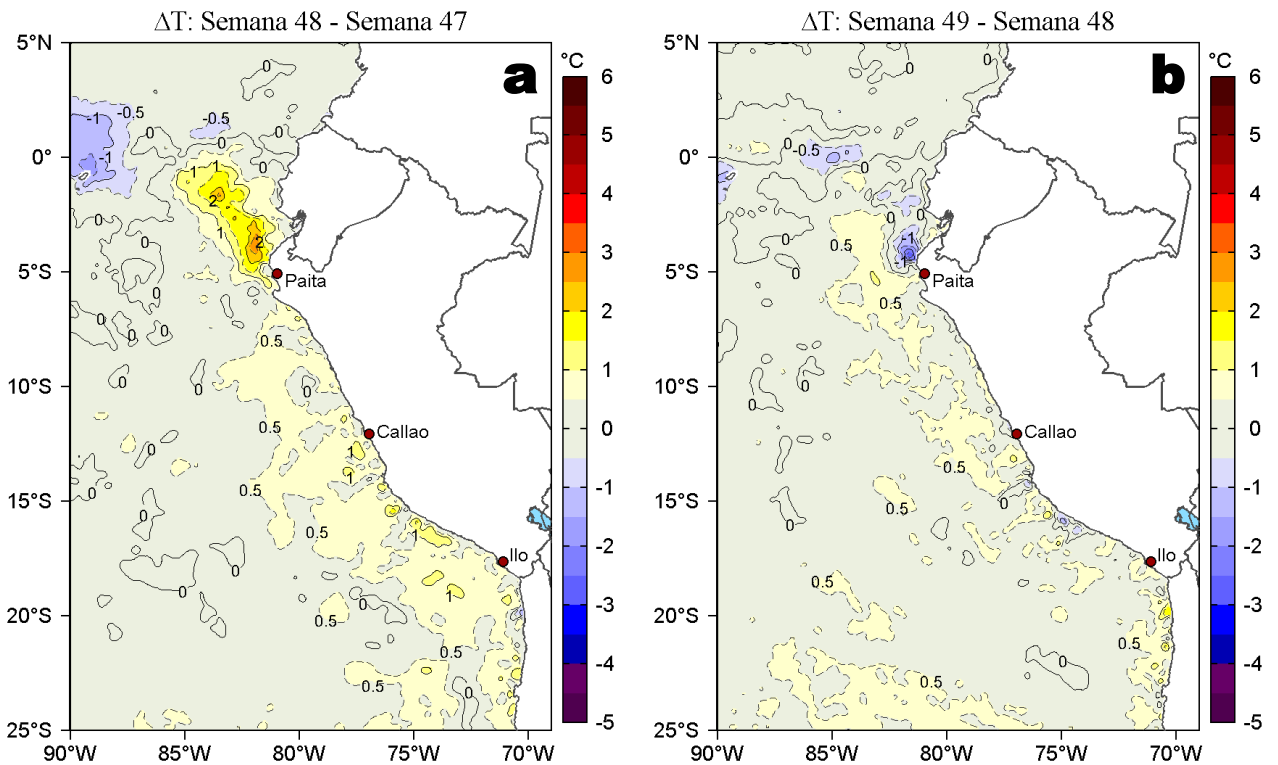
Figura 3. Variación semanal de la temperatura superficial del mar (°C) en el océano Pacífico tropical oriental entre: a) cuadragésima octava (26 de noviembre - 02 de diciembre) y cuadragésima séptima (19-25 de noviembre) semana de 2021 y b) cuadragésima novena (03-09 de diciembre) y cuadragésima octava (26 de noviembre - 02 de diciembre) semana de 2021. Los mapas, que indican el grado de calentamiento o enfriamiento de una semana a otra, provienen de OSTIA-UKMO-L4-GLOB-v2.0 (UK Met Office, 2012; Donlon et al, 2012). La barra de colores a la derecha muestra la diferencia de la temperatura entre la presente y la semana previa.
