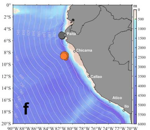
Figura 6. Diagrama Hovmöller de: a, d) Temperatura del mar (°C), b, d) Anomalías térmicas (°C) y c) Salinidad del mar de perfiladores ARGO localizados frente a Paita y Chicama los días 21 y 23 de noviembre, respectivamente. El primer flotador No. 6903002 se localizó a 41 mn (5,12 °S, 81,80 °W) de Paita mientras que el segundo (No. 3901808) se ubicó a 153 mn de Chicama (8,63 °S, 81,50 °W). Las anomalías de la temperatura del agua (°C) se calcularon de acuerdo a Domínguez et al (2017). Los puntos en la columna de agua indican los días en que los perfiladores registraron información. En la Figura (f) se muestra la ubicación de los perfiladores ARGO cuyos datos se han utilizado. Datos: ARGO.
