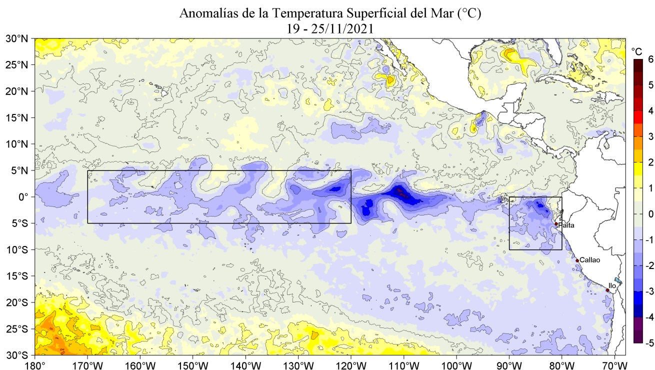
Figura 1. Anomalías promedio de la Temperatura superficial del mar ( ^{\circ}\text{C} ) en el océano Pacífico tropical para la semana del 19 al 25 de noviembre de 2021. Las regiones Niño 3.4 y Niño 1+2 en los sectores central y oriental del océano, respectivamente están delimitadas con una línea de color gris. Datos: OSTIA-UKMO-L4-GLOB-v2.0 (UK Met Office, 2012; Donlon et al, 2012) disponible en https://podaac.jpl.nasa.gov/dataset/OSTIA-UKMO-L4-GLOB-v2.0 . Las anomalías se calcularon con respecto de la climatología para el periodo 2007-2016.
