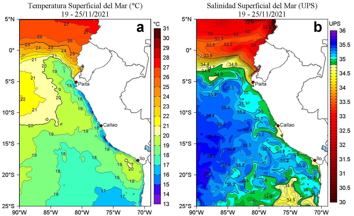
Figura 2. Distribución espacial promedio de: a) Temperatura (TSM, °C) y b) Salinidad superficial del mar (SSM) para la semana del 19 al 25 de noviembre de 2021, en el océano Pacífico oriental. Datos: OSTIA-UKMO-L4-GLOB-v2.0 (UK Met Office, 2012; Donlon et al, 2012) disponible en https://podaac.jpl.nasa.gov/dataset/OSTIA-UKMO-L4-GLOB-v2.0 para (a) y del GLOBAL ANALYSIS FORECAST PHY 001 024 (Lellouche, J. M. et al, 2013) disponible en http://marine.copernicus.eu/services-portfolio/access-to-products/?option=com_csw&view=details&product_id=GLOBAL_ANALYSIS_FORECAST_PHY_001_024 para (b). Las escalas de colores se presentan a la derecha de cada gráfico.
