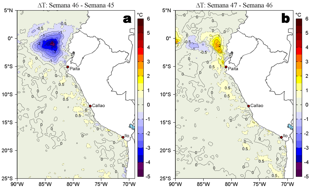
Figura 3. Variación semanal de la temperatura superficial del mar (°C) en el océano Pacífico tropical oriental entre: a) cuadragésima sexta (12-18 de noviembre) y cuadragésima quinta (05-11 de noviembre) semana de 2021 y b) cuadragésima séptima (19-25 de noviembre) y cuadragésima sexta (12-18 de noviembre) semana de 2021. Los mapas, que indican el grado de calentamiento o enfriamiento de una semana a otra, provienen de OSTIA-UKMO-L4-GLOB-v2.0 (UK Met Office, 2012; Donlon et al, 2012). La barra de colores a la derecha muestra la diferencia de la temperatura entre la presente y la semana previa.
