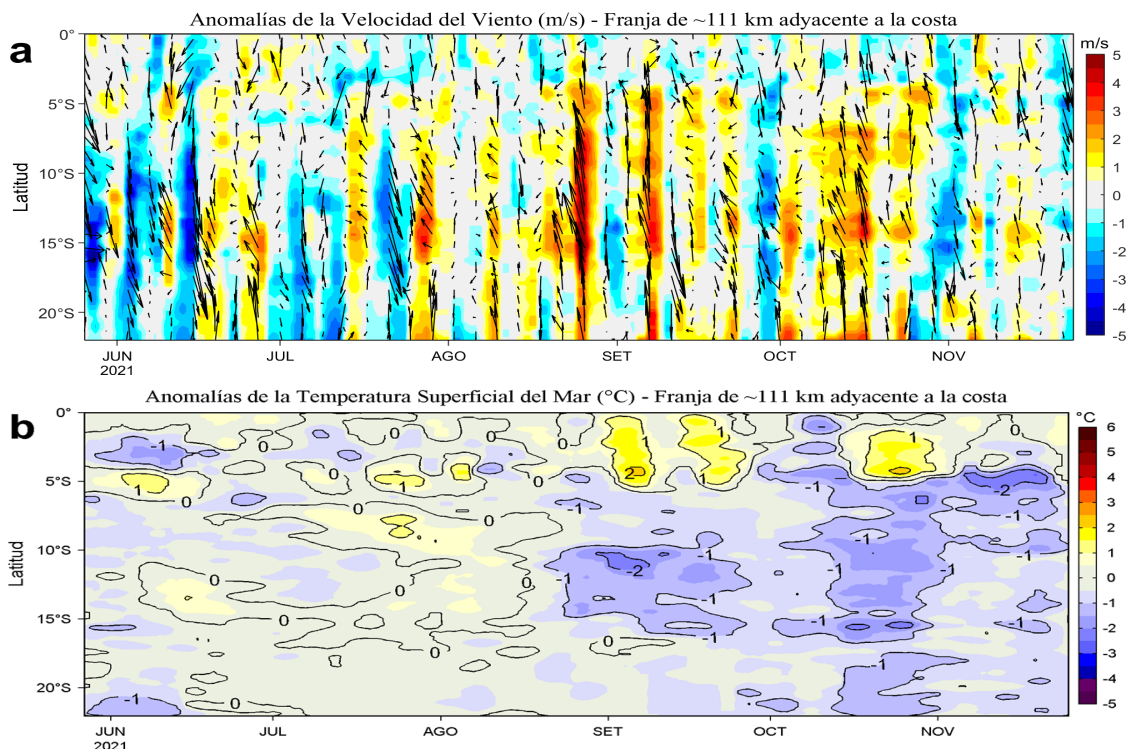
Figura 4. Evolución de las anomalías diarias de: a) Velocidad del viento (m/s) y b) Temperatura superficial del mar (°C) para el último semestre, actualizado al 24 y 25 de noviembre de 2021, respectivamente. Datos: de IFREMER/CERSAT para (a) y de OSTIA-UKMO-L4-GLOB-v2.0 para (b). Las anomalías fueron calculadas para una franja de 111 km adyacente a la costa entre el ecuador geográfico y 22°S según los promedios climatológicos diarios de 2000-2014 para (a) y de 2007-2016 para (b). La barra de colores a la derecha muestra la escala de las anomalías en cada caso.
