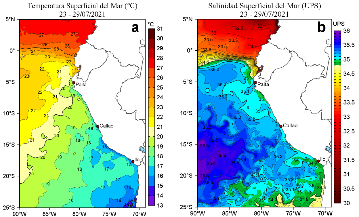
Figura 2. Distribución espacial promedio de: a) Temperatura (TSM, °C) y b) Salinidad superficial del mar (SSM) para la semana del 23 al 29 de julio de 2021, en el océano Pacífico oriental. Datos: OSTIA-UKMO-L4-GLOB-v2.0 (UK Met Office, 2012; Donlon et al, 2012) disponible en https://podaac.jpl.nasa.gov/dataset/OSTIA-UKMO-L4-GLOB-v2.0 para (a) y del GLOBAL_ANALYSIS_FORECAST_PHY_001_024 (Lellouche, J. M. et al, 2013) disponible en http://marine.copernicus.eu/services-portfolio/access-to-products/?option=com_csw&view=details&product_id=GLOBAL_ANALYSIS_FORECAST_PHY_001_024 para (b). Las escalas de colores se presentan a la derecha de cada gráfico.
