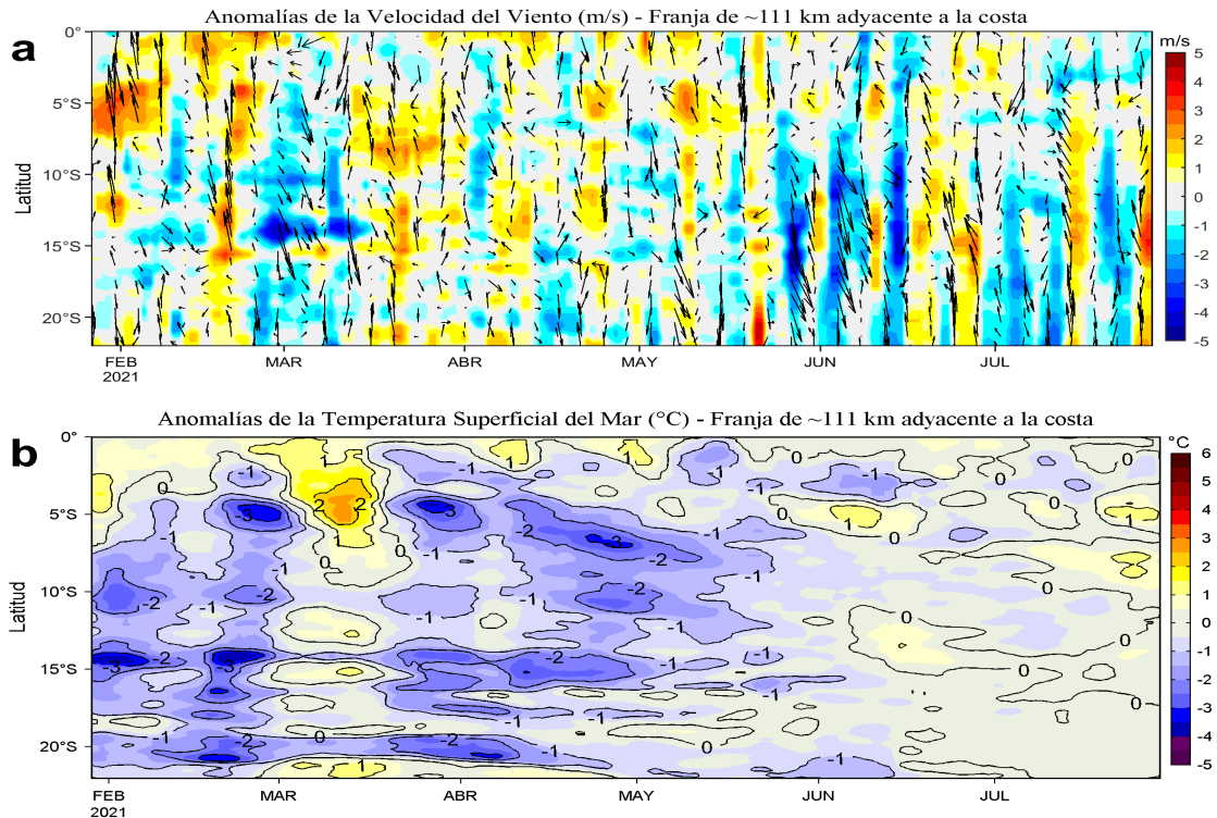
Figura 4. Evolución de las anomalías diarias de: a) Velocidad del viento (m/s) y b) Temperatura superficial del mar (°C) para el último semestre, actualizado al 28 y 29 de julio de 2021, respectivamente. Datos: de IFREMER/CERSAT para (a) y de OSTIA-UKMO-L4-GLOB-v2.0 para (b). Las anomalías fueron calculadas para una franja de 111 km adyacente a la costa entre el ecuador geográfico y 22°S según los promedios climatológicos diarios de 2000-2014 para (a) y de 2007-2016 para (b). La barra de colores a la derecha muestra la escala de las anomalías en cada caso.
