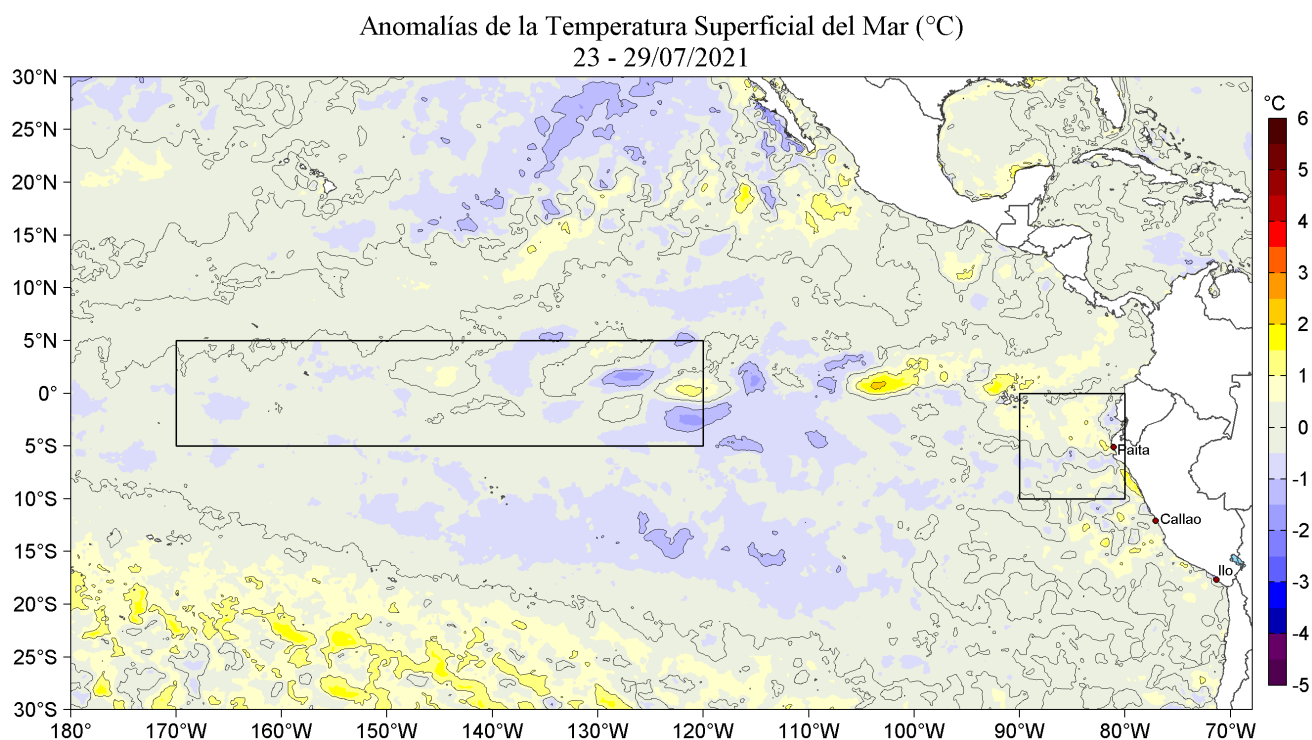
Figura 1. Anomalías promedio de la Temperatura superficial del mar ( ^{\circ}\text{C} ) en el océano Pacífico tropical para la semana del 23 al 29 de julio de 2021. Las regiones Niño 3.4 y Niño 1+2 en los sectores central y oriental del océano, respectivamente están delimitadas con una línea de color gris. Datos: OSTIA-UKMO-L4-GLOB-v2.0 (UK Met Office, 2012; Donlon et al, 2012) disponible en https://podaac.jpl.nasa.gov/dataset/OSTIA-UKMO-L4-GLOB-v2.0 . Las anomalías se calcularon con respecto de la climatología para el período 2007-2016.
