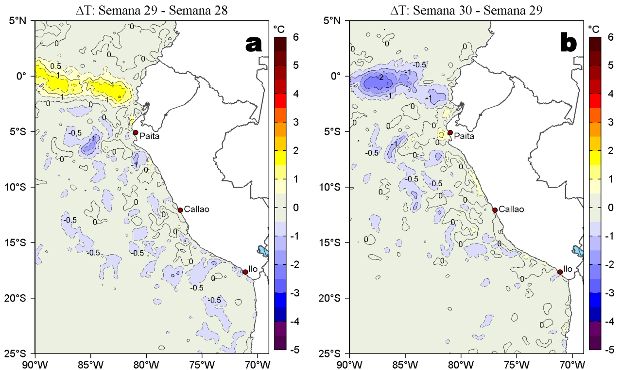
Figura 3. Variación semanal de la temperatura superficial del mar (°C) en el océano Pacífico tropical oriental entre: a) vigésima novena (16-22 de julio) y vigésima octava (09-15 de julio) semana de 2021 y b) trigésima (23-29 de julio) y vigésima novena (16-22 de julio) semana de 2021. Los mapas, que indican el grado de calentamiento o enfriamiento de una semana a otra, provienen de OSTIA-UKMO-L4-GLOB-v2.0 (UK Met Office, 2012; Donlon et al, 2012). La barra de colores a la derecha muestra la diferencia de la temperatura entre la presente y la semana previa.
