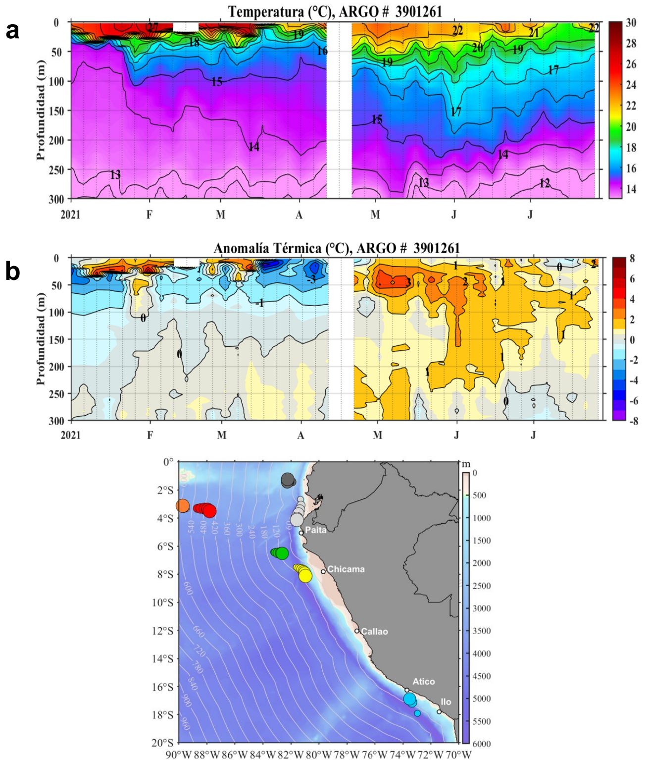
Figura 6. Diagrama Hovmöller de: a) Temperatura del mar (°C) y b) Anomalías térmicas (°C) del perfilador ARGO No. 3901261 localizado a 27 millas (4,14°S y 81,57°W) frente a Piura del 01 de enero al 26 de julio de 2021. Las anomalías de la temperatura del agua (°C) se calcularon de acuerdo a Domínguez et al (2017). Los puntos en la columna de agua indican los días en que el perfilador ARGO registró información. En la Figura (c) se muestra la ubicación de los perfiladores ARGO disponibles en el área de estudio. La ubicación del perfilador ARGO No. 3901261 se presenta con el círculo de color gris claro. Datos: ARGO.
