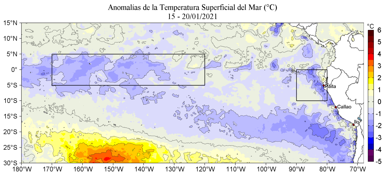
Figura 1. Anomalías promedio de la Temperatura superficial del mar (°C) en el océano Pacífico tropical para la semana del 15 al 20 de enero de 2021. Las regiones Niño 3.4 y Niño 1+2 en los sectores central y oriental del océano, respectivamente están delimitadas con una línea de color gris. Datos: OSTIA-UKMO-L4-GLOB-v2.0 (UK Met Office, 2012; Donlon et al, 2012) disponible en https://podaac.jpl.nasa.gov/dataset/OSTIA-UKMO-L4-GLOB-v2.0 . Las anomalías se calcularon con respecto de la climatología para el período 2007-2016.
