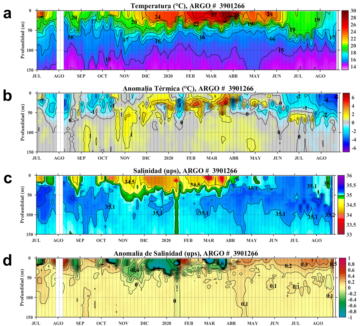
Figura 5. Diagrama Hovmöller de: a) Temperatura del mar (°C), b) Anomalías térmicas (°C), c) Salinidad del agua de mar (ups) y d) Anomalía de la salinidad del mar (ups) a 270 mn frente a Tumbes (~85°W y ~2,8°S) de julio del 2019 al 23 de agosto de 2020. Las anomalías de la temperatura del agua (°C) y de salinidad (ups) se calcularon de acuerdo a Domínguez et al (2017). Los puntos en la columna de agua indican los días en que el perfilador ARGO registró información. Datos: ARGO. Procesamiento: LHQM/AFIOQ/DGIOCC/IMARPE.
