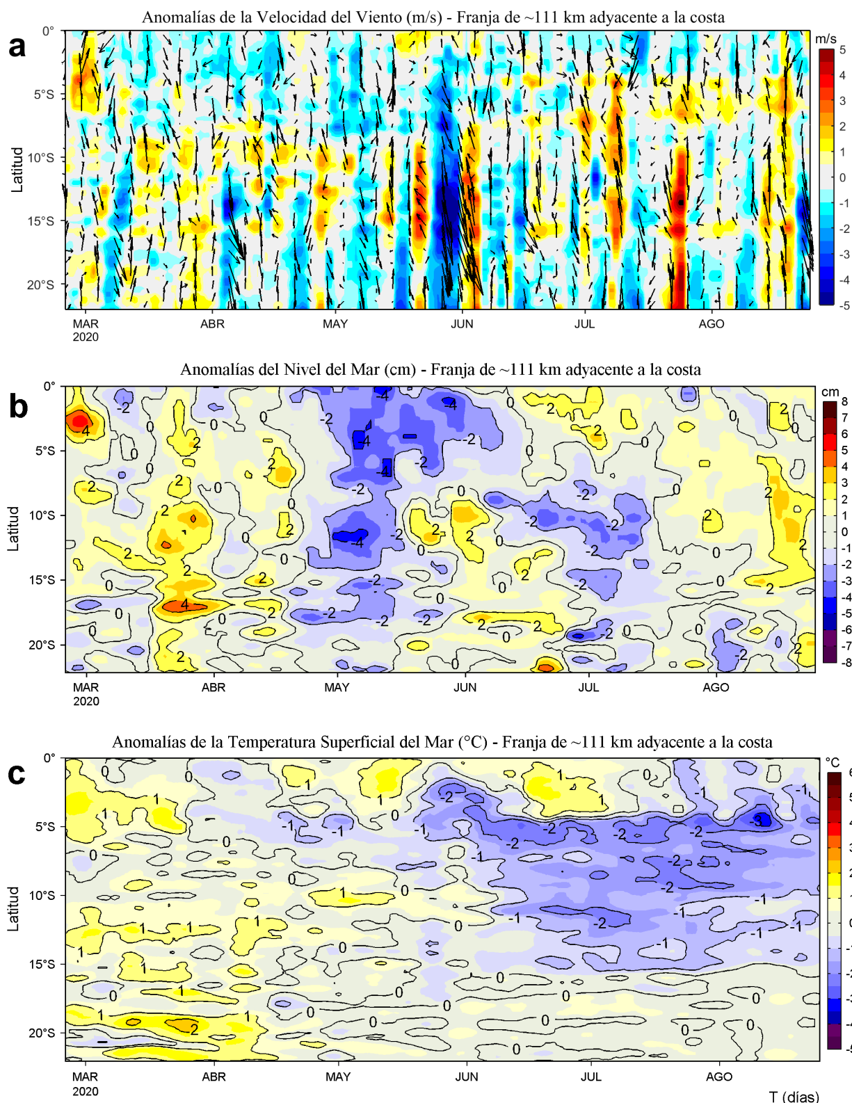
Figura 4. Evolución de las anomalías diarias de: a) Velocidad del viento (m/s), b) Nivel del mar (cm), c) Temperatura superficial del mar (°C) para el último semestre, actualizado al 25 de agosto de 2020. Los datos de anomalías de nivel del mar consideran un filtro pasa alto de 120 días. Datos: de IFREMER/CERSAT para (a), del Servicio de Monitoreo del Ambiente Marino Copernicus (CMEMS en inglés) para (b), de OSTIA-UKMO-L4-GLOB-v2.0 para (c). Las anomalías fueron calculadas para una franja de 111 km adyacente a la costa entre el ecuador y 22°S según los promedios climatológicos diarios de 2000-2014 para (a), de 1993-2010 para (b) y de 2007-2016 para (c). La barra de colores a la derecha muestra la escala de las anomalías en cada caso. Procesamiento: LHFm/AFIOF/DGIOCC/IMARPE.
