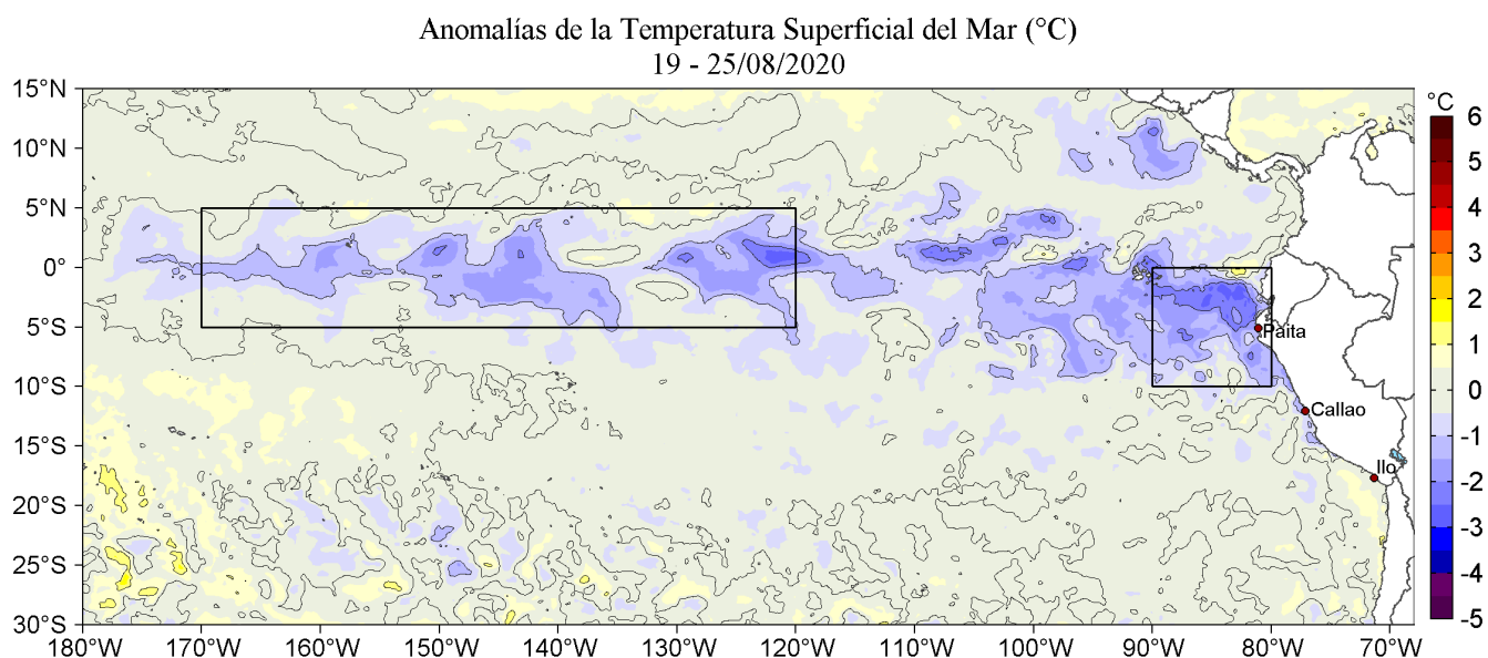
Figura 2. Anomalías promedio de la Temperatura superficial del mar (°C) en el océano Pacífico tropical para la semana del 19 al 25 de agosto de 2020. Las regiones Niño 3.4 y Niño 1+2 en los sectores central y oriental del océano, respectivamente están delimitadas con una línea de color gris. Datos: OSTIA-UKMO-L4-GLOB-v2.0 (UK Met Office, 2012; Donlon et al, 2012) disponible en https://podaac.jpl.nasa.gov/dataset/OSTIA-UKMO-L4-GLOB-v2.0 . Las anomalías se calcularon con respecto de la climatología para el período 2007-2016. Procesamiento: LHFm/AFIOF/DGIOCC/IMARPE.
