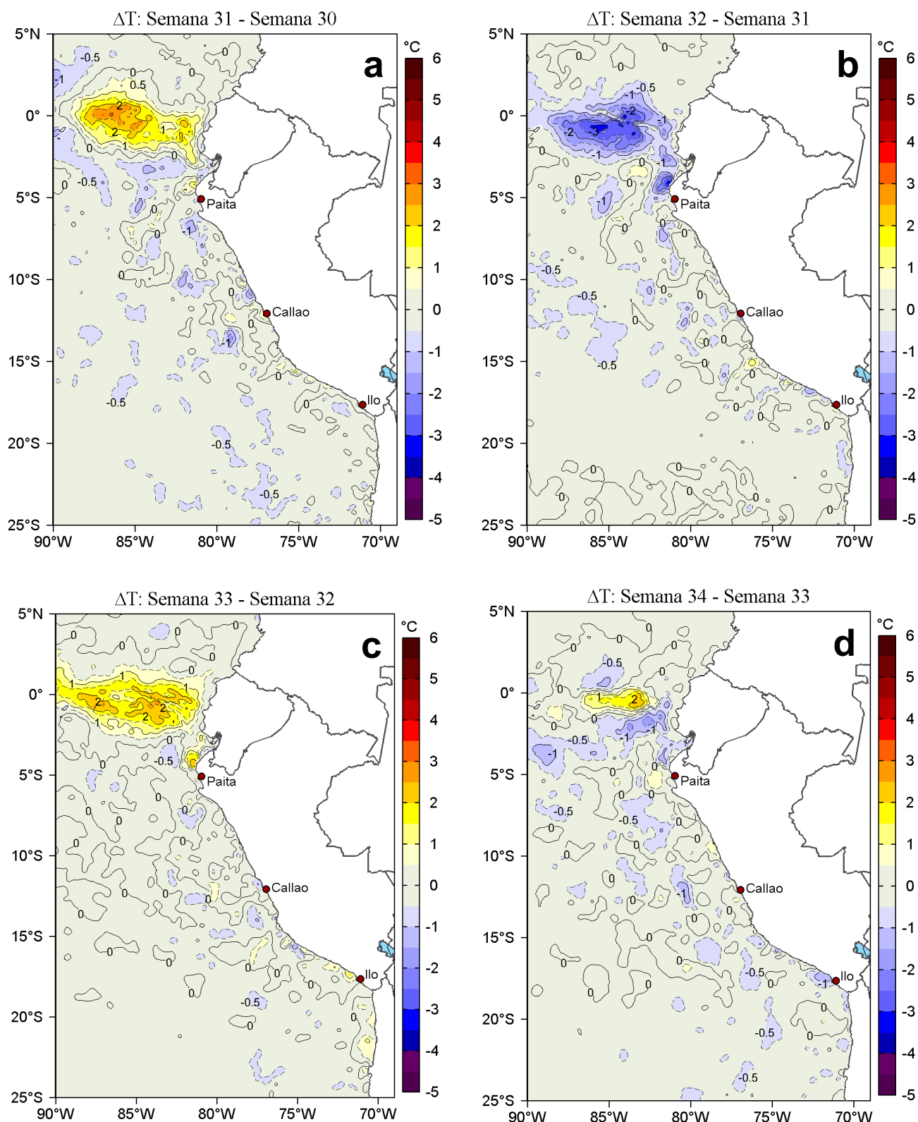
Figura 3. Variación semanal de la temperatura superficial del mar (°C) en el océano Pacífico tropical oriental entre: a) trigésima primera (29 de julio - 04 de agosto) y trigésima (22-28 de julio) semana del 2020, b) trigésima segunda (05-11 de agosto) y trigésima primera (29 de julio - 04 de agosto) semana del 2020, c) trigésima tercera (12-18 de agosto) y trigésima segunda (05-11 de agosto) semana del 2020 y d) trigésima cuarta (19-25 de agosto) y trigésima tercera (12-18 de agosto) semana del 2020. Los mapas, que indican el grado de calentamiento o enfriamiento de una semana a otra, provienen de OSTIA-UKMO-L4-GLOB-v2.0 (UK Met Office, 2012; Donlon et al, 2012). La barra de colores a la derecha muestra la diferencia de la temperatura entre la presente y la semana previa. Procesamiento: LHFm/AFIOF/DGIOCC/IMARPE.
