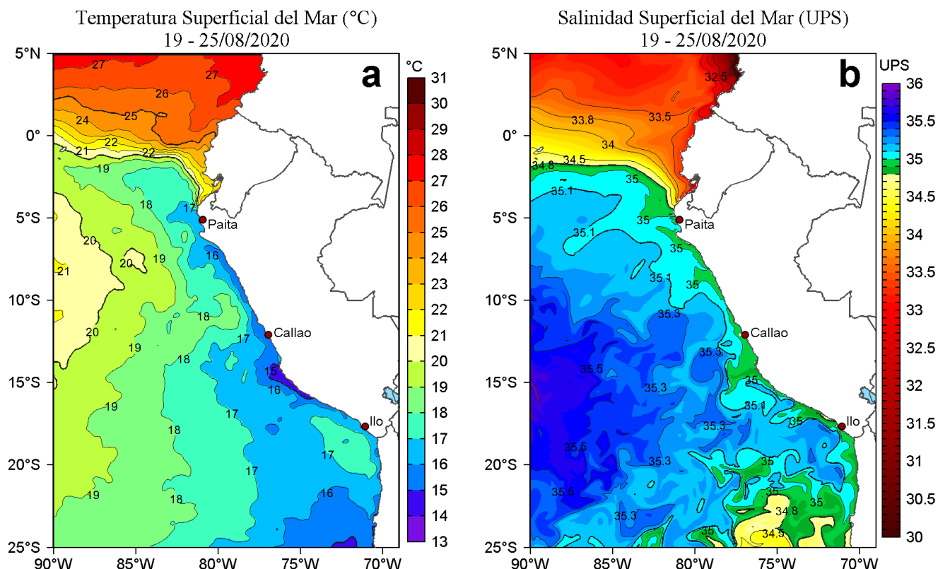
Figura 1. Distribución espacial promedio de: a) Temperatura superficial del mar (TSM, °C) y b) Salinidad superficial del mar (SSM, ups) para la semana del 19 al 25 de agosto de 2020 en el océano Pacífico tropical oriental. Datos: OSTIA-UKMO-L4-GLOB-v2.0 (UK Met Office, 2012; Donlon et al, 2012) disponible en https://podaac.jpl.nasa.gov/dataset/OSTIA-UKMO-L4-GLOB-v2.0 para (a) y del GLOBAL_ANALYSIS_FORECAST_PHY_001_024 (Lellouche, J.-M. et al, 2013) disponible en http://marine.copernicus.eu/services-portfolio/access-to-products/?option=com_csw&view=details&product_id=GLOBAL_ANALYSIS_FORECAST_PHY_001_024 para (b). Las escalas de colores de la TSM como de la SSM se presentan a la derecha de cada gráfico. Procesamiento: LHFm/AFIOF/DGIOCC/IMARPE.
