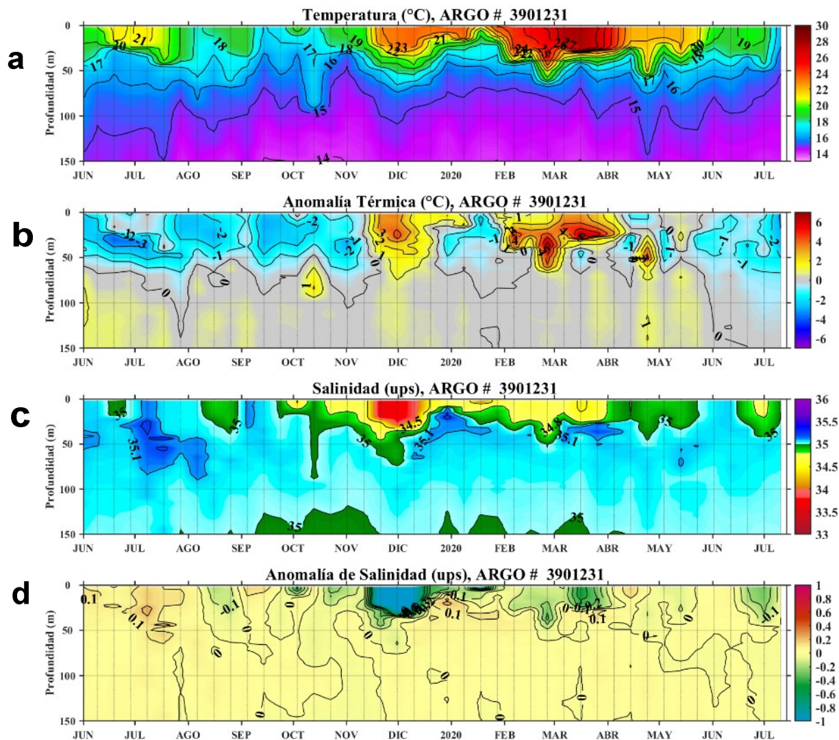
Figura 5. Diagrama Hovmöller de: a) Temperatura del mar (°C), b) Anomalías térmicas (°C), c) Salinidad del agua de mar (ups) y d) Anomalía de la salinidad del mar (ups) frente a Talara (~82,2°W y ~4,4°S) de junio del 2019 al 10 de julio de 2020. Las anomalías de la temperatura del agua (°C) y de salinidad (ups) se calcularon de acuerdo a Domínguez et al (2017). Los puntos en la columna de agua indican los días en que el perfilador ARGO registró información. Datos: ARGO. Procesamiento: LHQM/AFIOQ/DGIOCC/IMARPE.
