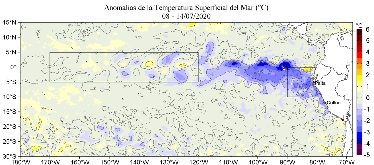
Figura 2. Anomalías promedio de la Temperatura superficial del mar (°C) en el océano Pacífico tropical para la semana del 08 al 14 de julio de 2020. Las regiones Niño 3.4 y Niño 1+2 en los sectores central y oriental del océano, respectivamente están delimitadas con una línea de color gris. Datos: OSTIA-UKMO-L4-GLOB-v2.0 (UK Met Office, 2012; Donlon et al, 2012) disponible en https://podaac.jpl.nasa.gov/dataset/OSTIA-UKMO-L4-GLOB-v2.0 . Las anomalías se calcularon con respecto de la climatología para el período 2007-2016. Procesamiento: LHF/AFIOF/DGIOCC/IMARPE.
