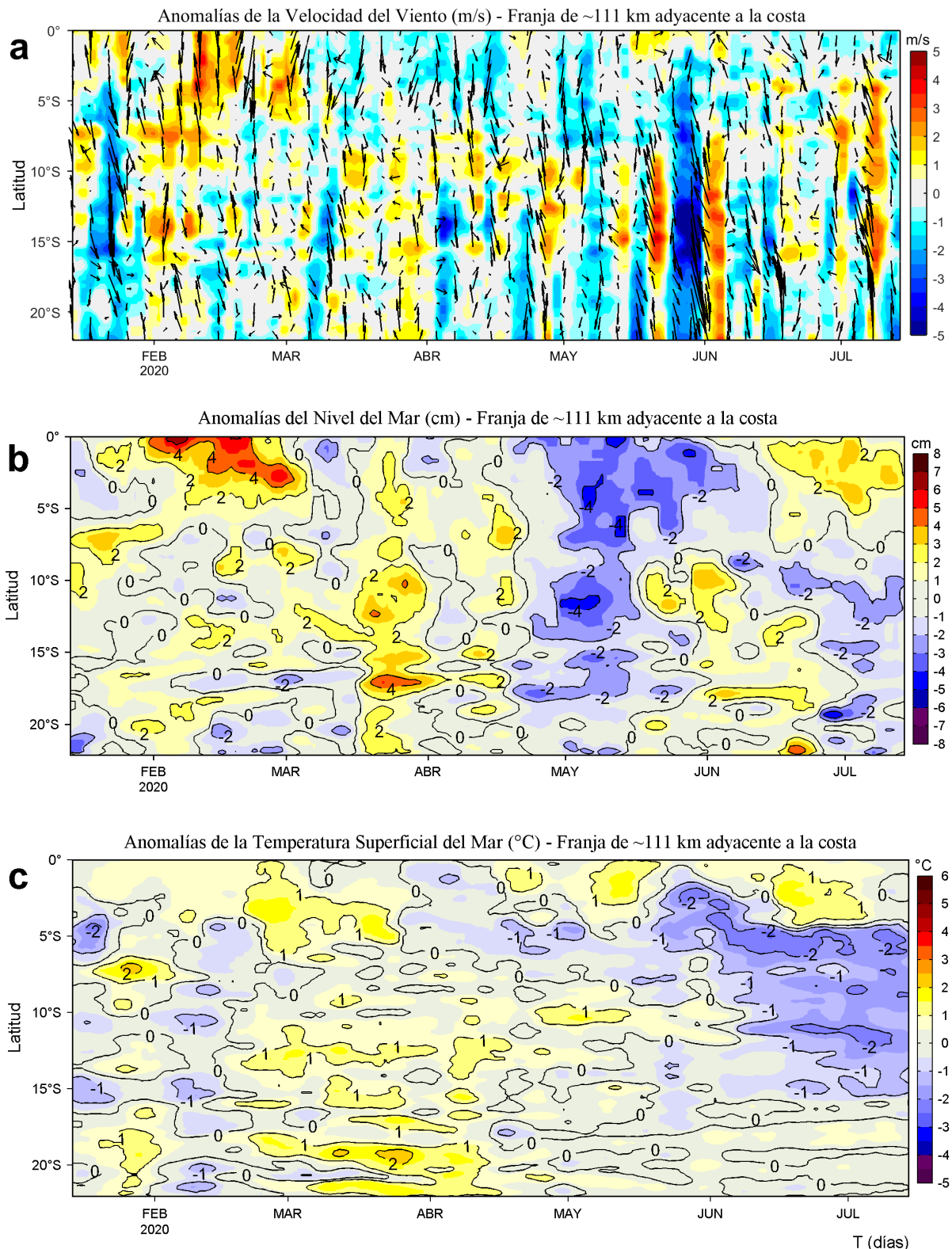
Figura 4. Evolución de las anomalías diarias de: a) Velocidad del viento (m/s), b) Nivel del mar (cm), c) Temperatura superficial del mar (°C) para el último semestre, actualizado al 14 de julio de 2020. Los datos de anm consideran un filtro pasa alto de 120 días. Datos: de IFREMER/CERSAT para (a), del Servicio de Monitoreo del Ambiente Marino Copernicus (CMEMS en inglés) para (b), de OSTIA-UKMO-L4-GLOB-v2.0 para (c). Las anomalías fueron calculadas para una franja de 111 km adyacente a la costa entre el ecuador y 22°S según los promedios climatológicos diarios de 2000-2014 para (a), de 1993-2010 para (b) y de 2007-2016 para (c). La barra de colores a la derecha muestra la escala de las anomalías en cada caso. Procesamiento: LHF/AFIOF/DGIOCC/IMARPE.
