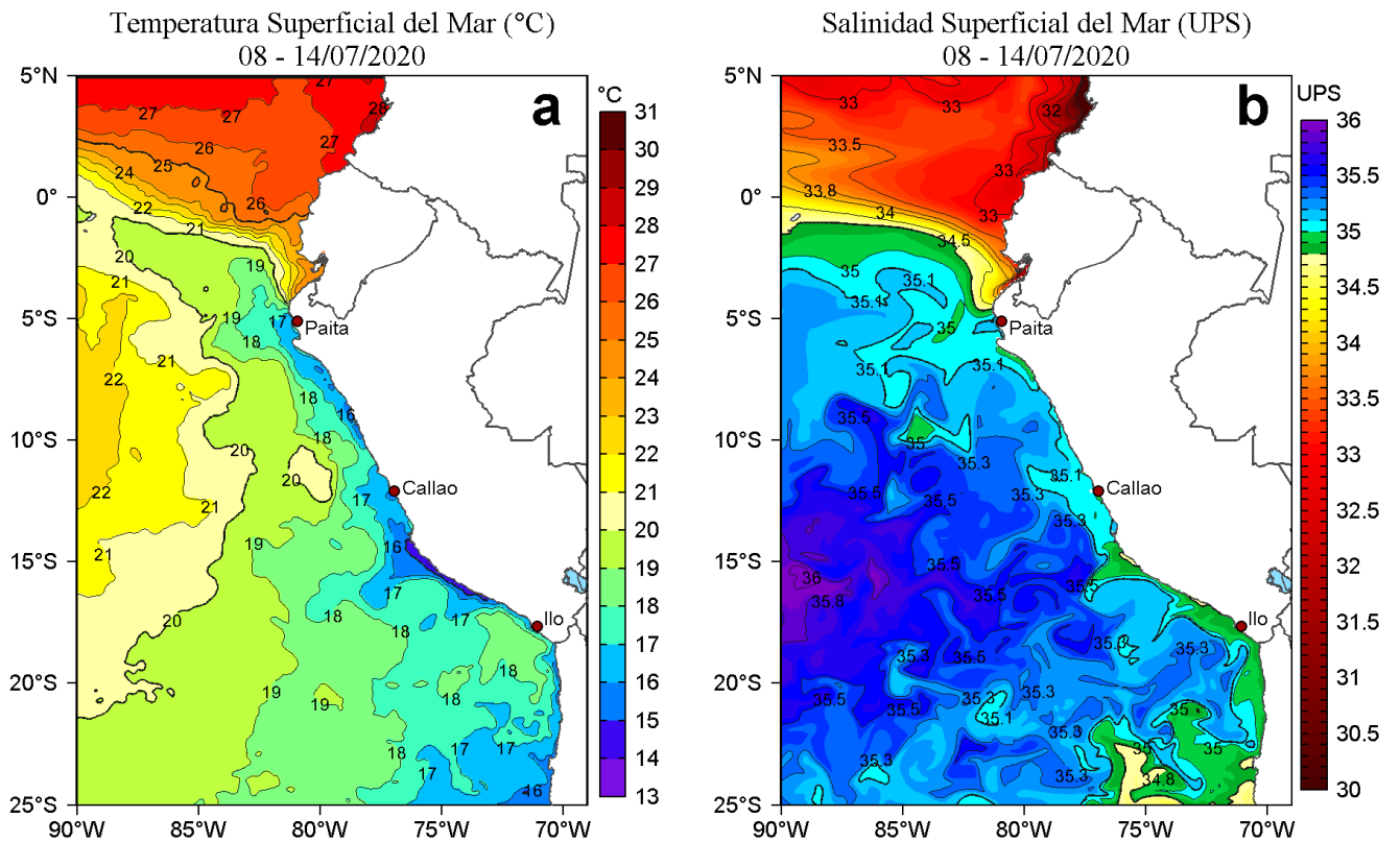
Figura 1. Distribución espacial promedio de: a) Temperatura superficial del mar (TSM, °C) y b) Salinidad superficial del mar (SSM, ups) para la semana del 08 al 14 de julio de 2020 en el océano Pacífico tropical oriental. Datos: OSTIA-UKMO-L4-GLOB-v2.0 (UK Met Office, 2012; Donlon et al, 2012) disponible en https://podaac.jpl.nasa.gov/dataset/OSTIA-UKMO-L4-GLOB-v2.0 para (a) y del GLOBAL_ANALYSIS_FORECAST_PHY_001_024 (Lellouche, J.-M. et al, 2013) disponible en http://marine.copernicus.eu/services-portfolio/access-to-products/?option=com_csw&view=details&product_id=GLOBAL_ANALYSIS_FORECAST_PHY_001_024 para (b). Las escalas de colores de la TSM como de la SSM se presentan a la derecha de cada gráfico. Procesamiento: LHF/AFIOF/DGIOCC/IMARPE.
