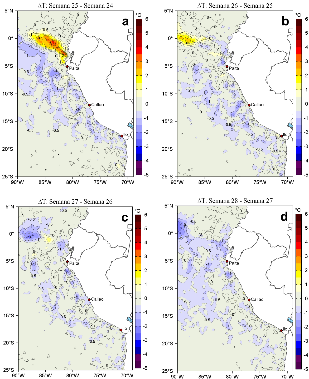
Figura 3. Variación semanal de la temperatura superficial del mar ( ^{\circ}\text{C} ) en el océano Pacífico tropical oriental entre: a) vigésima quinta (17-23 de junio) y vigésima cuarta (10-16 de junio) semana del 2020, b) vigésima sexta (24-30 de junio) y vigésima quinta (17-23 de junio) semana del 2020, c) vigésima séptima (01-07 de julio) y vigésima sexta (24-30 de junio) semana del 2020 y d) vigésima octava (08-14 de julio) y vigésima séptima (01-07 de julio) semana del 2020. Los mapas, que indican el grado de calentamiento o enfriamiento de una semana a otra, provienen de OSTIA-UKMO-L4-GLOB-v2.0 (UK Met Office, 2012; Donlon et al, 2012). La barra de colores a la derecha muestra la diferencia de la temperatura entre la presente y la semana previa. Procesamiento: LHF/AFIOF/DGIOCC/IMARPE.
